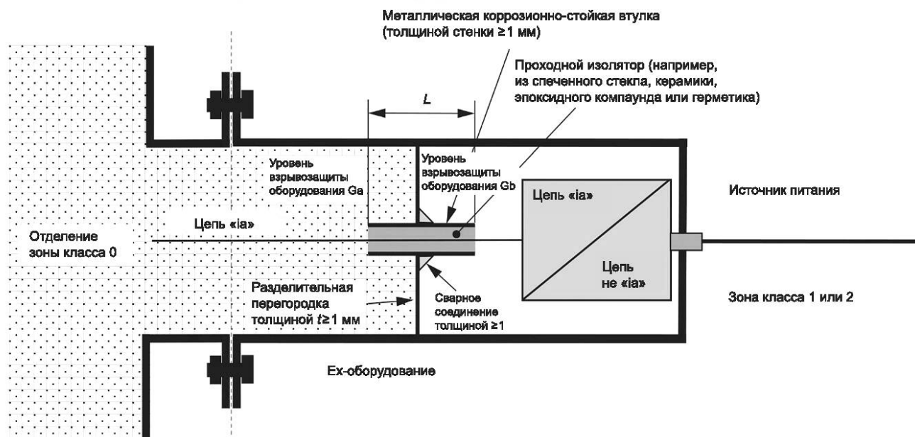
Рисунок 1 — Пример газонепроницаемой разделительной перегородки с проходным изолятором
