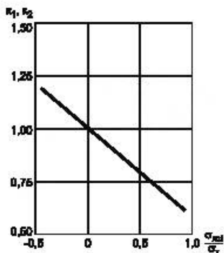
Рисунок А.1 — Диаграмма зависимости коэффициентов k_1, k_2 от значения относительной величины суммарных средних напряжений \frac{\sigma_m}{\sigma_T}
