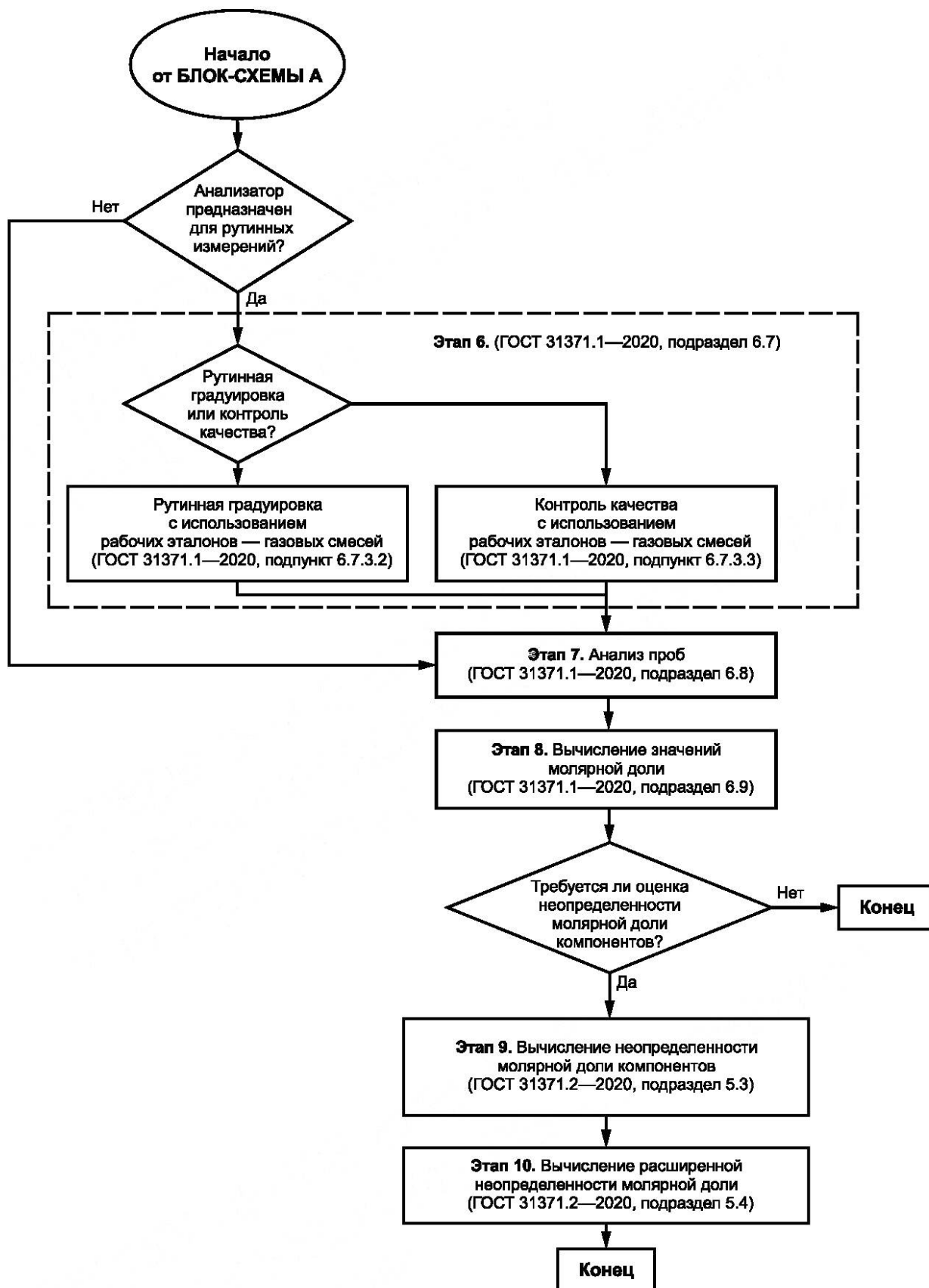
Рисунок 2 — Процедура определения молярной доли и неопределенности — этапы 6—10 (блок-схема В)
