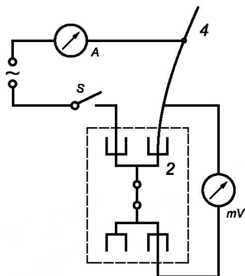
б) принципиальная схема для определения падения напряжения во время испытаний на изгиб винтовых контактных зажимов
