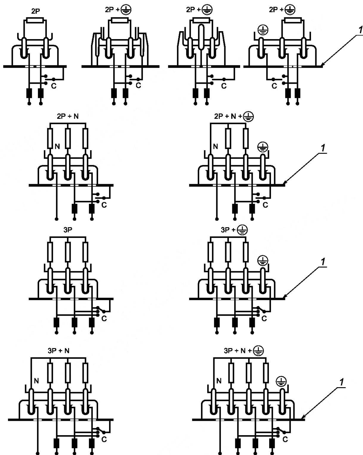
Рисунок 17 — Схема соединения для испытания на нормальную работу
