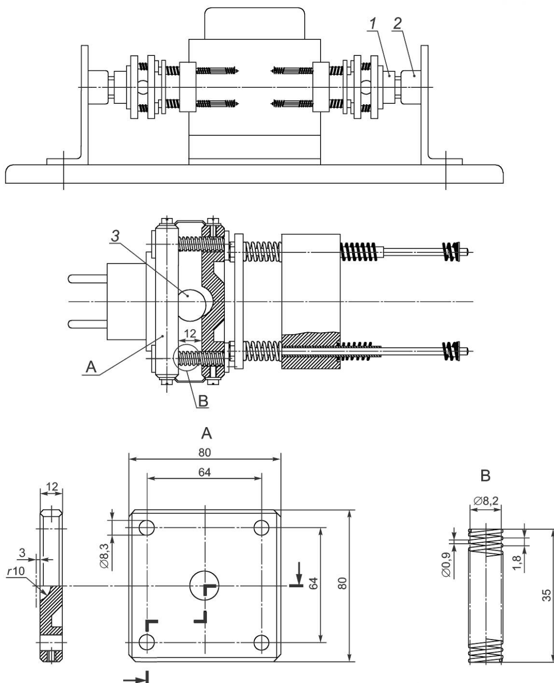
1 — вилка; 2 — розетка; 3 — стальной шар
