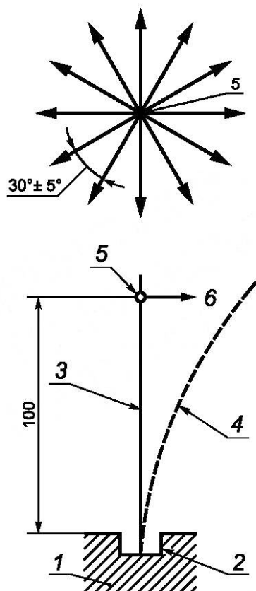
а) принцип действия испытательной установки для проверки на изгиб безвинтовых контактных зажимов
