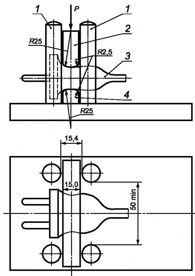
Рисунок 38 — Установка для испытания на сжатие вилок
