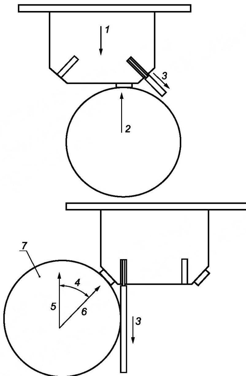
b) испытательная установка
