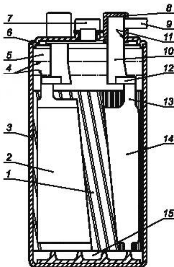
1 – сепаратор; 2 – положительно заряженная пластина; 3 – контейнер элемента; 4 – уровень электролита (макс./мин.); 5 – свободное пространство; 6 – уплотнение, непроницаемое для электролита; 7 – втулка для залива и слива; 8 – герметизированная оболочка держателя; 9 – соединитель между элементами; 10 – держатель вывода; 11 – уплотнение держателя, непроницаемое для электролита; 12 – стержень; 13 – опора пластины; 14 – отрицательно заряженная пластина; 15 – пространство для конденсата.
