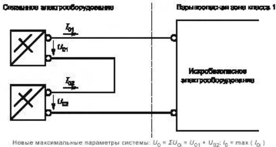
Рисунок В.1 – Последовательное соединение. Суммирование напряжений
