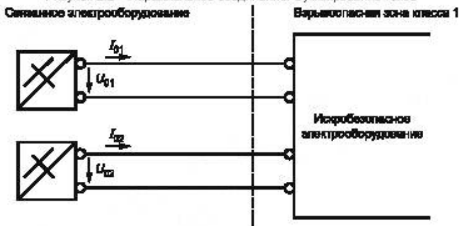
Рисунок В.2 – Параллельное соединение. Суммирование токов
