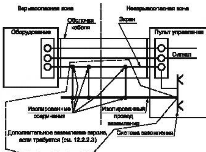
Рисунок 2 - Заземление проводящих экранов
