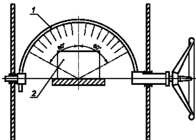
1 — трубка; 2 — образец
