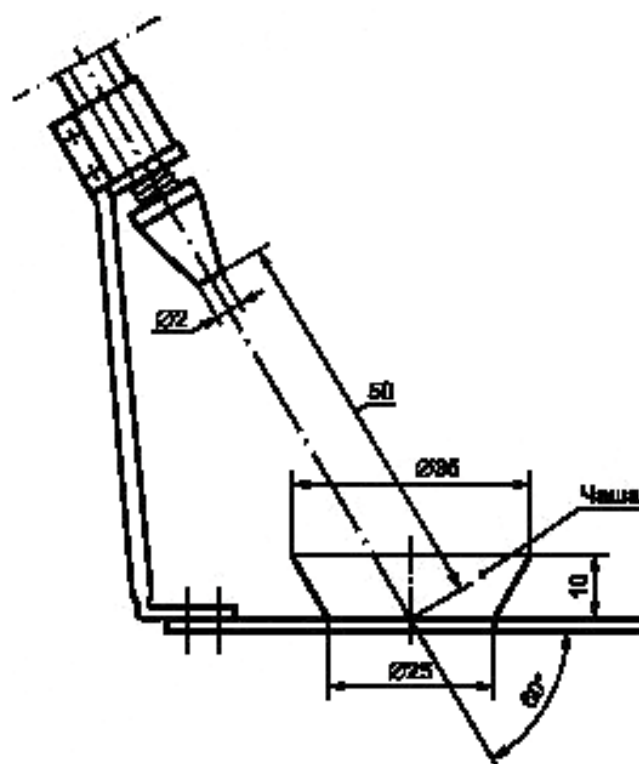
Рисунок 4 — Разбрызгиватель
