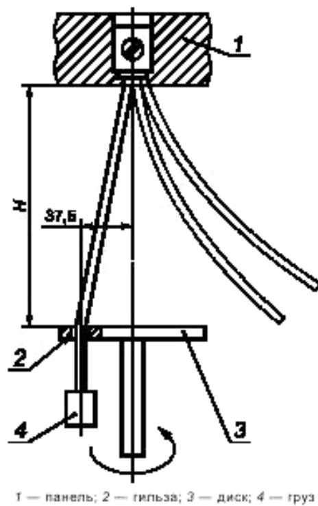
Рисунок 15 — Установка для испытаний проводников на изгиб
