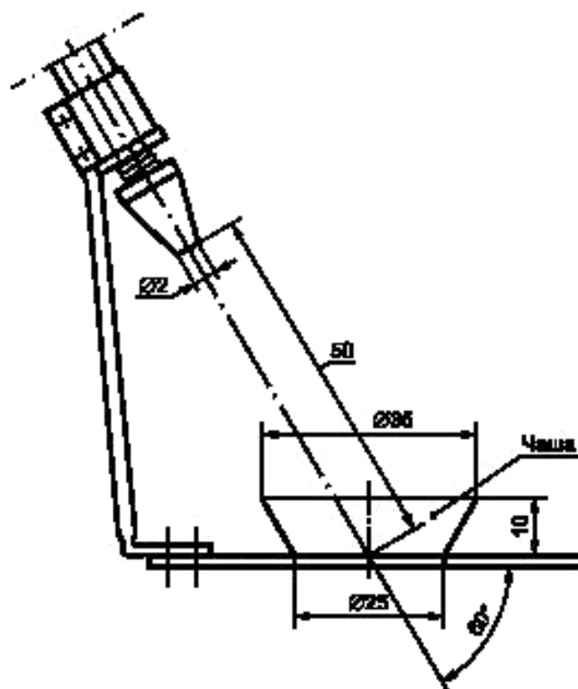
Рисунок 4 — Разбрызгиватель
