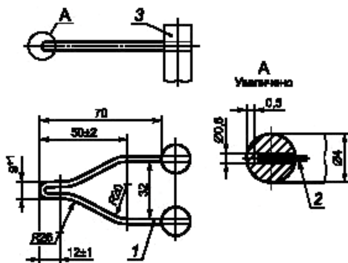
1 — раскаленная петля, запаиваемая в стойки; 2 — термопара; 3 — стойка
