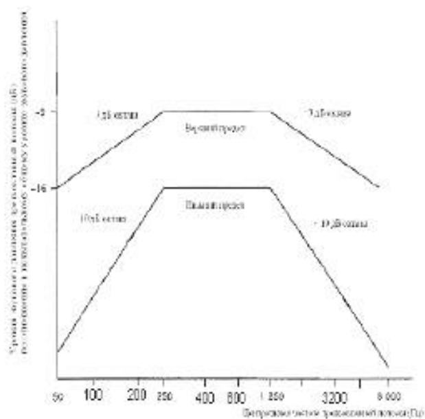
Рисунок 1 – Спектр частотной характеристики для аудионаушников
