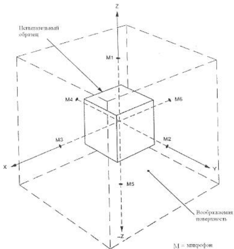
Рисунок 5 - Типовое расположение микрофонов контрольных точек (1-6) на вообразаемой поверхности вокруг образца
