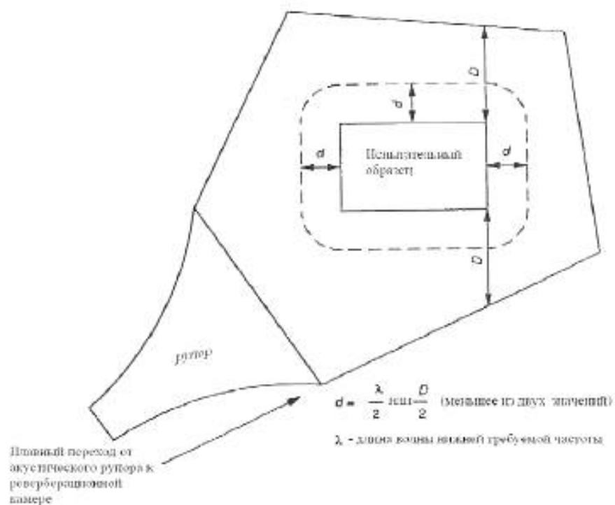
Рисунок 4 - Типовое расположение микрофонов вокруг образца
