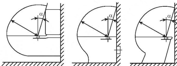
Рисунок 1 — Расположение отверстий под крепления сиденья
