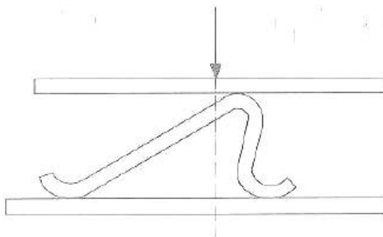
Рисунок 3 – Наклон гофров
