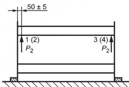
Рисунок 2 — Схема нагружения верхнего яруса кровати
