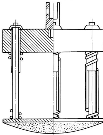
Рисунок Б.1 — Ударное устройство
