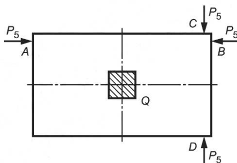
Рисунок 4 — Схема нагружения кровати
