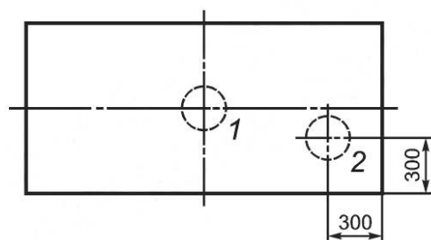
Рисунок 6 — Расположение точек нагружения основания кровати
