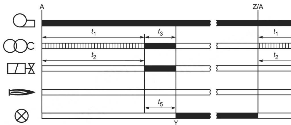
Рисунок СС.6 — Выключение питания вследствие невосстановления сигнала пламени (в течение времени защитного отключения t_5 )
