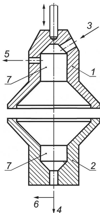
1 — верхняя секция (подвижная); 2 — нижняя секция (фиксированная); 3 — входное отверстие для контрольного аэрозоля; 4 — выходное отверстие для контрольного аэрозоля; 5 — зона отбора проб до фильтра; 6 — зона отбора проб после фильтра; 7 — точки измерения перепада давления
