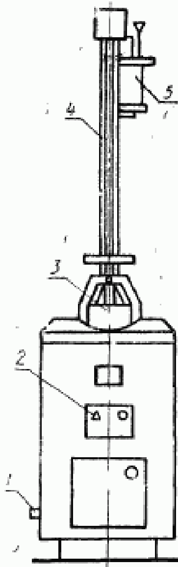
1 — водосливной кран; 2 — рукоятка; 3 — испытательная головка; 4 — манометр; 5 — сосуд Мариотта
