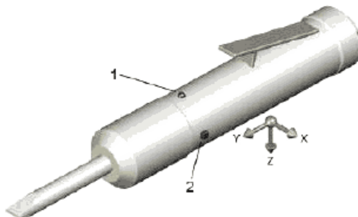
Рисунок 5 – Точки и направления измерений для прямого молотка
