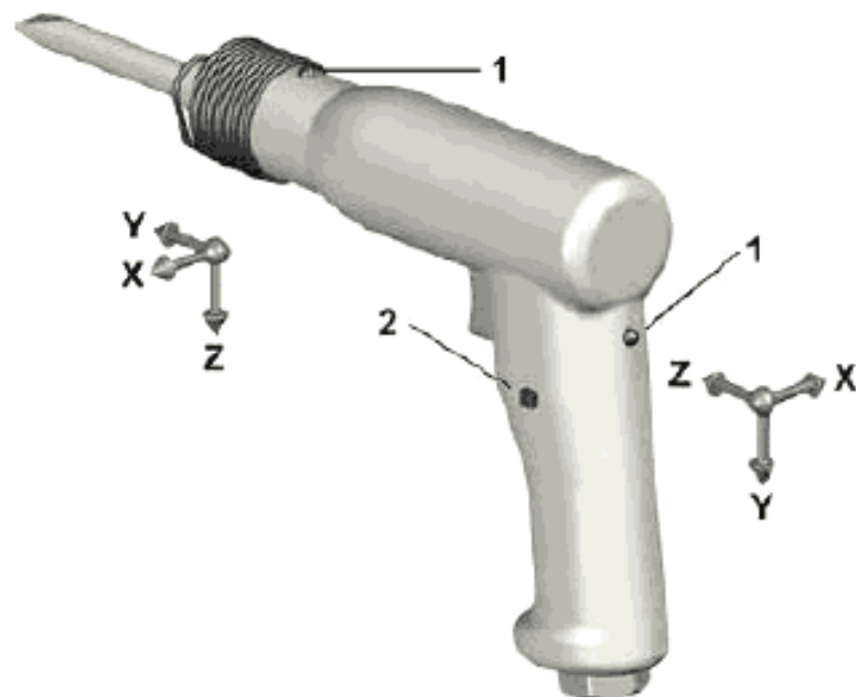
Рисунок 7 – Точки и направления измерений для молотка с рукояткой пистолетного типа
