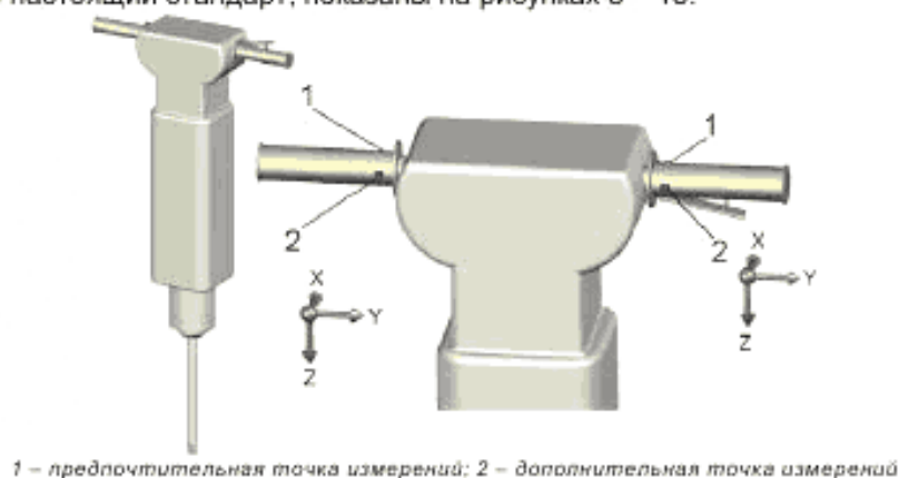
Рисунок 8 – Лом / бурильный молоток
