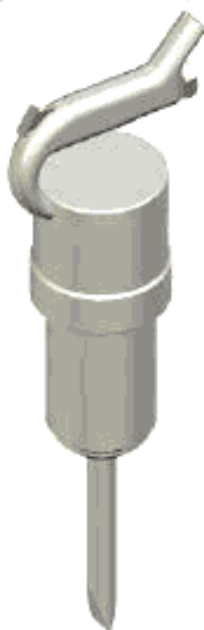
Рисунок 3 – Большой обрубочный молоток / перфоратор для анкерных работ
