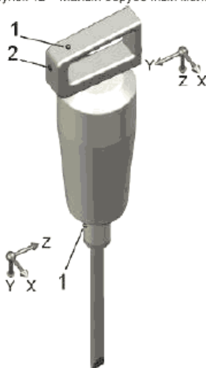
Рисунок 13 – Отбойный молоток
