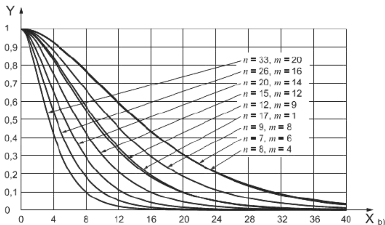
Рисунок 2 – Кривые оперативных характеристик для планов контроля доли несоответствующих единиц продукции с \alpha \leq 5\% и \beta \leq 10\%
