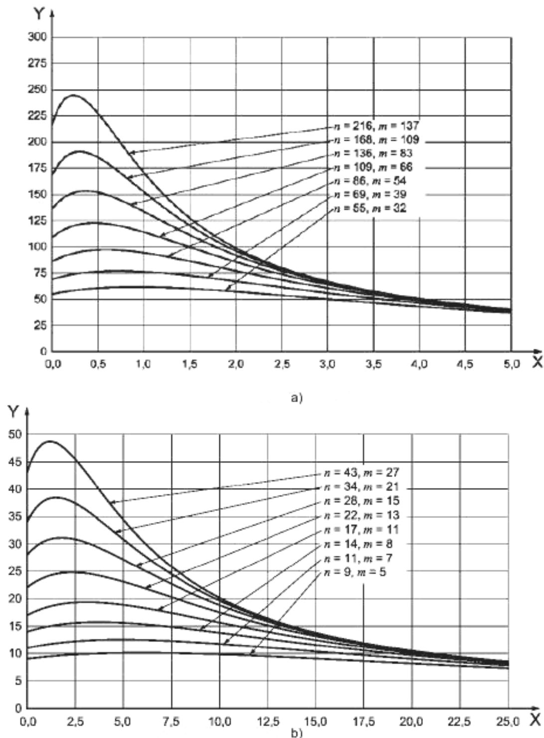
Рисунок 23 – Кривая среднего объема выборки для планов контроля числа несоответствий, усеченный контроль с \alpha \leq 5\% и \beta \leq 10\%
