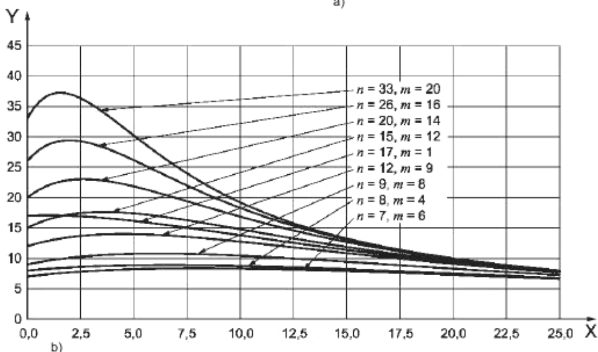
Рисунок 20 – Кривые среднего объема выборки для планов контроля доли несоответствующих единиц продукции, усеченный контроль с \alpha \leq 5\% и \beta \leq 10\%
