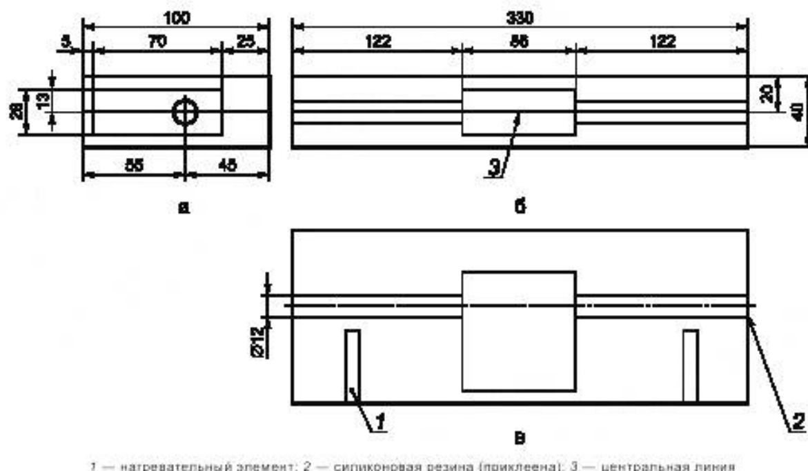
Рисунок 2 — Алюминиевая обогреваемая камера
