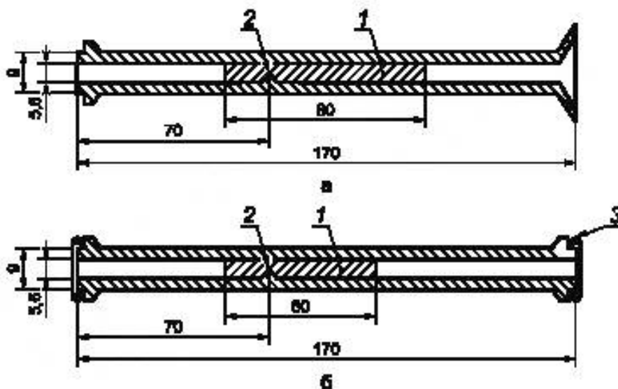
1 — нить из сплава золото/платина; 2 — выступ; 3 — уплотнительное кольцо
