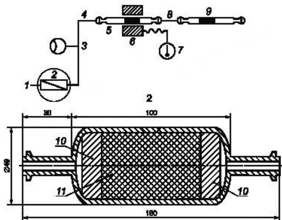
1 — воздушный насос; 2 — ловушка для ртути; 3 — ротаметр; 4 — трубки из ПВА; 5 — проботборная трубка; 6 — печь для трубок; 7 — термометр; 8 — соединительная стеклянная трубка; 9 — аналитическая трубка; 10 — стекловолокно; 11 — адсорбент (например, активированный уголь, обработанный серой)
