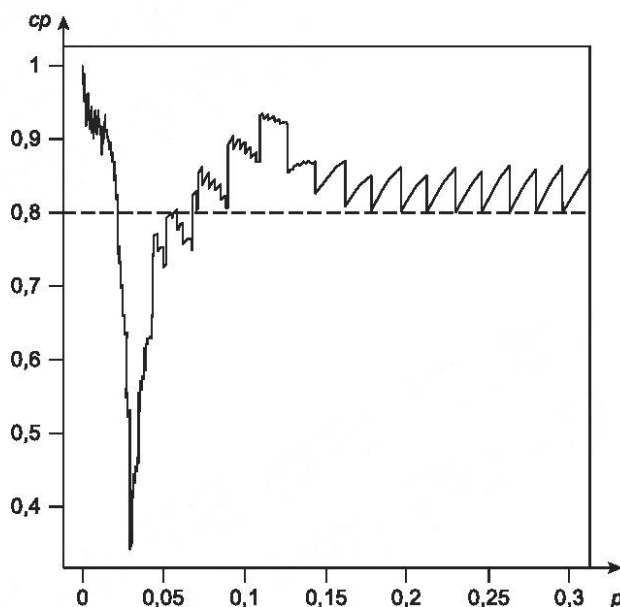
Рисунок G.1 — Фактическая вероятность охвата в примере 1 [при среднем уровне показателя доверия, номинальном значении доверительной вероятности \gamma = 0,80 и допустимой доле несоответствующих единиц p_0 = 0,03 , график сгенерирован для параметров (Trust = «Mid», gamma = 0,80, p_0 = 0,03 , p_capped = TRUE)]
