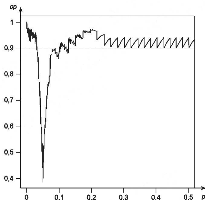
Рисунок G.5 — Фактическая вероятность охвата в примере 5 [при среднем уровне показателя доверия, номинальном уровне доверительной вероятности \gamma = 0,90 и допустимой доле несоответствующих единиц p_0 = 0,05 , график сгенерирован для параметров (Trust = «Mid», gamma = 0,90, p_0 = 0,05 , p_capped = TRUE)]
