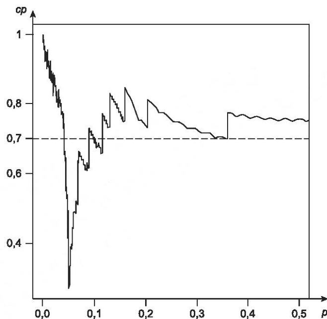
Рисунок G.4 — Фактическая вероятность охвата в примере 4 [при низком уровне показателя доверия, номинальном уровне доверительной вероятности \gamma = 0,70 и допустимой доле несоответствующих единиц p_0 = 0,05 , график сгенерирован для параметров (Trust = «Low», gamma = 0,70, p_0 = 0,05 , p_capped = TRUE)]
