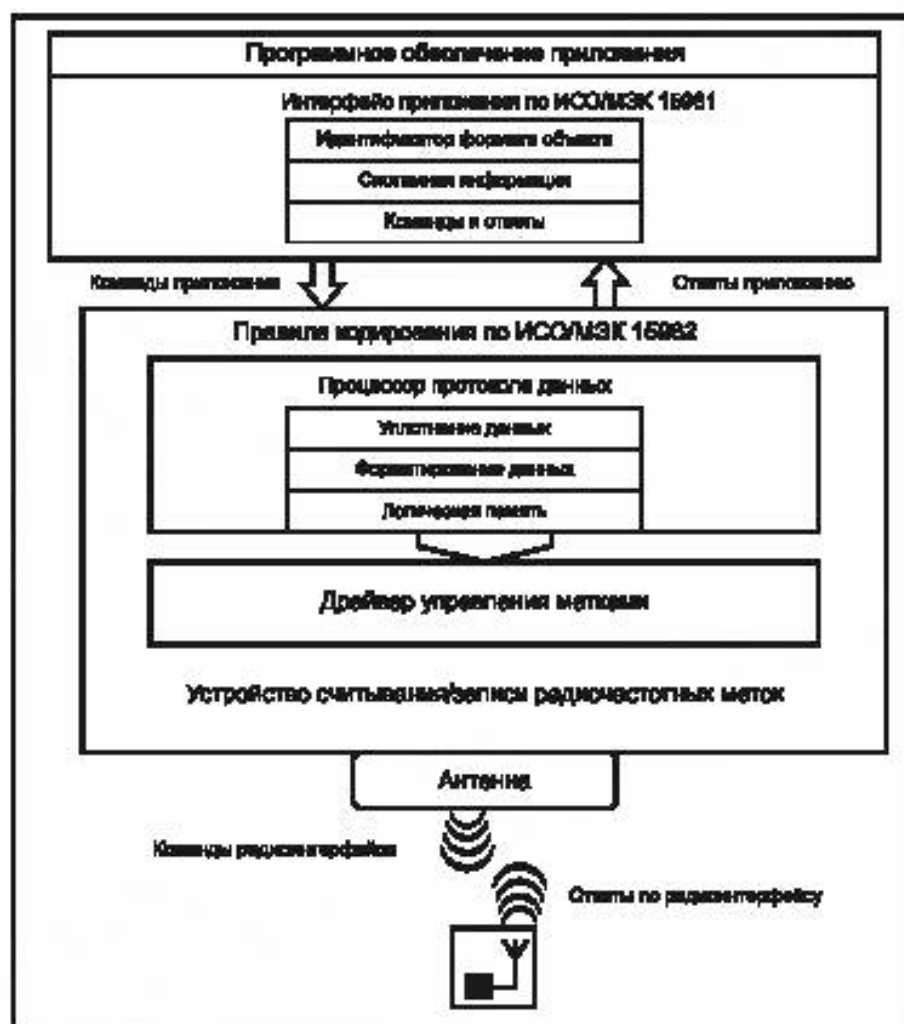
Рисунок 3 — Архитектура протокола данных радиочастотной идентификации по ИСО
