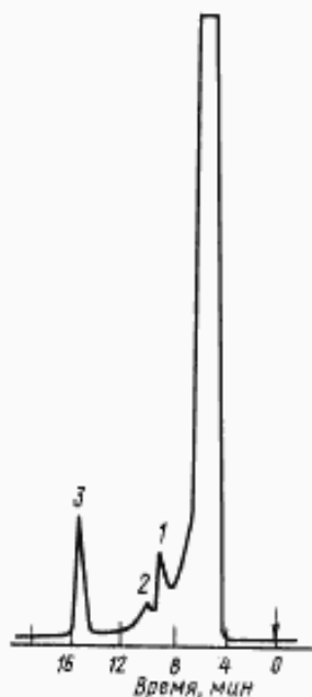
Типовая хроматограмма технического ацетона
