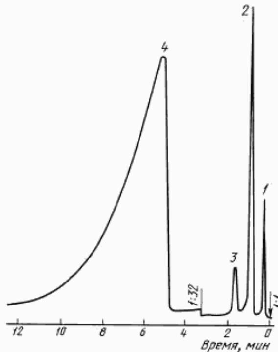
Типовая хроматограмма анализа ацетона
