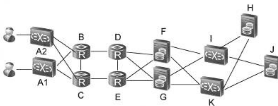
Рисунок В.1 — Пример типичной топологии сети в целом
