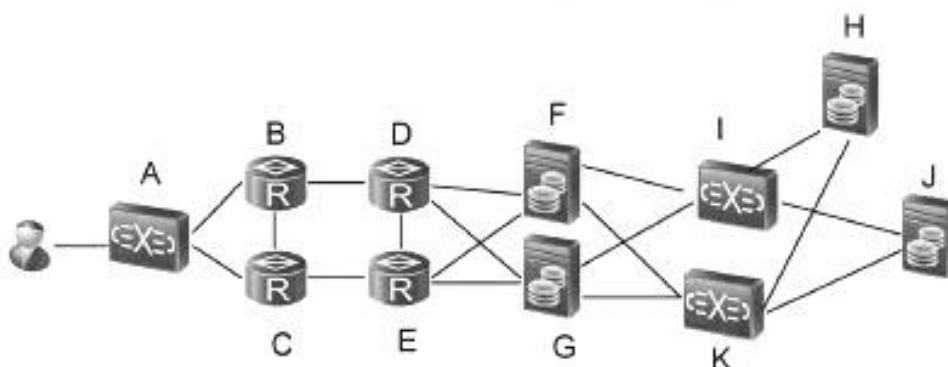
Рисунок А.1 — Пример типичной топологии сети E2E
