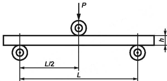
Рисунок 2 — Схема испытания образца
