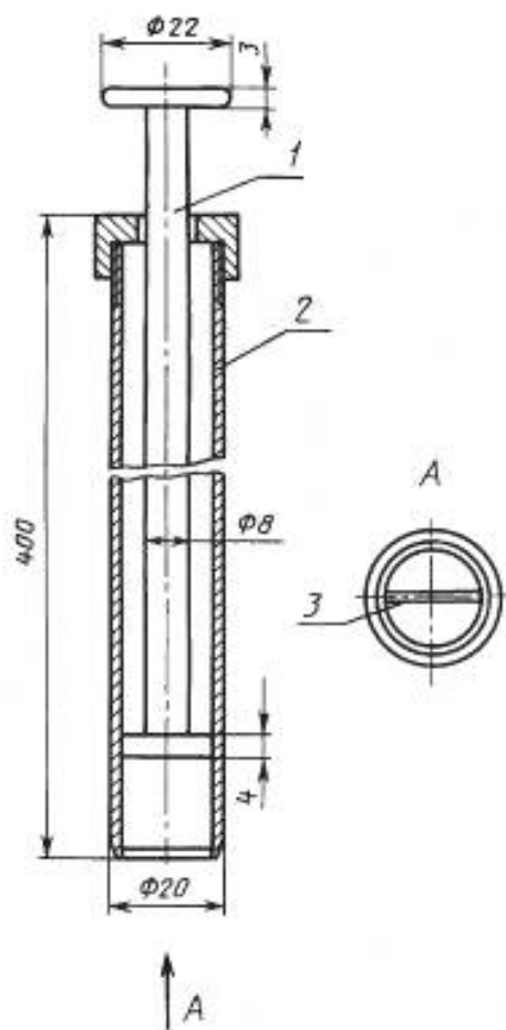
Поршневой щуп
