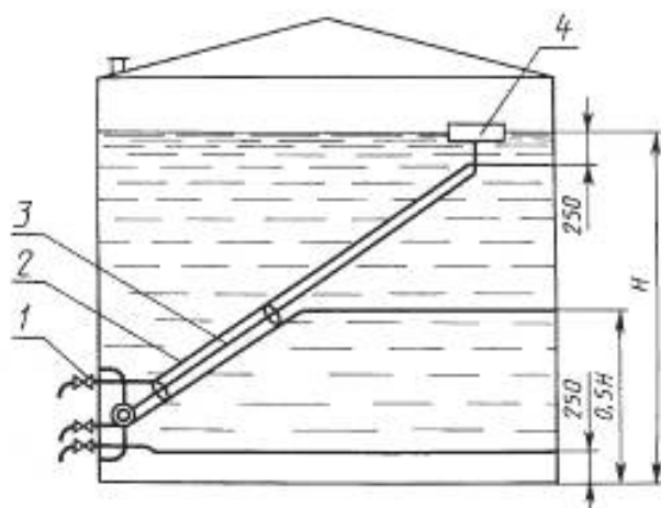
1 — кран; 2 — пробозаборные трубки; 3 — несущий рычаг; 4 — поплавок
