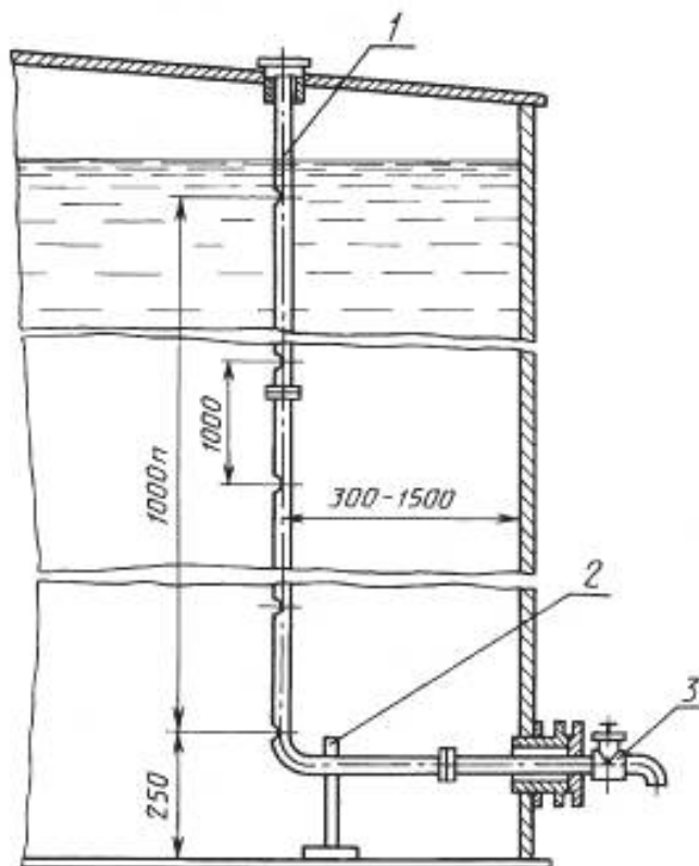
1 — перфорированная заборная трубка; 2 — опорная стойка; 3 — кран
