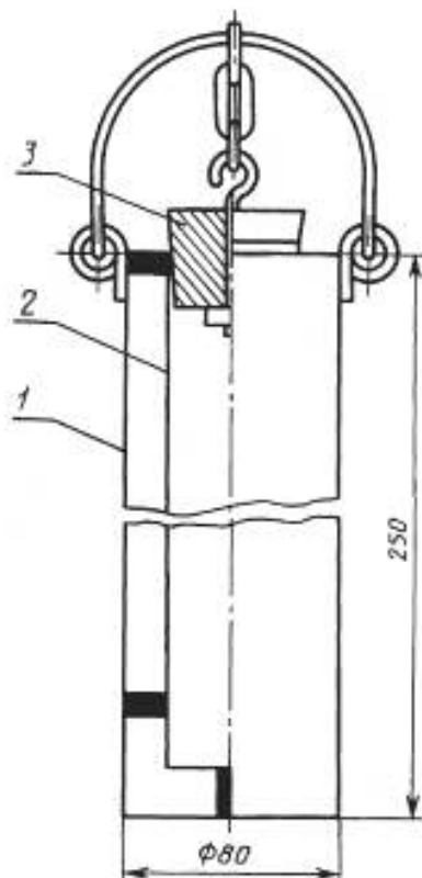
Термостатический пробоотборник
