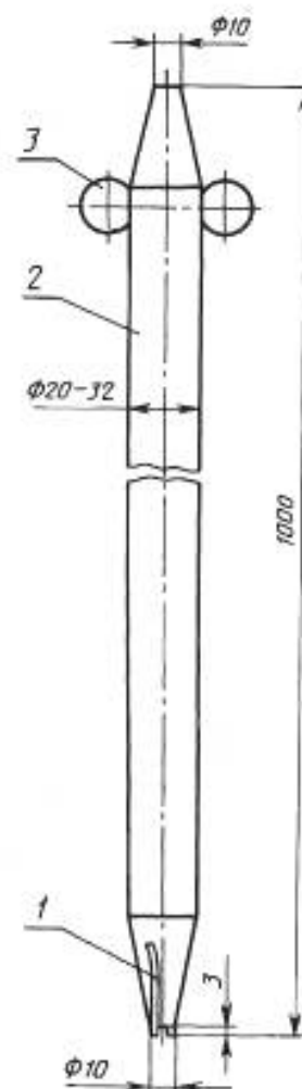
Пробоотборная трубка
