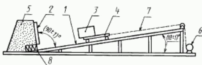
Схема наклонной плоскости
