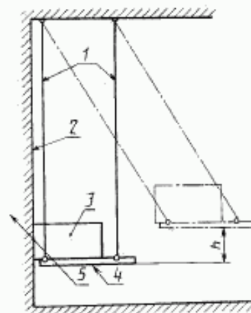
Схема маятникового прибора
