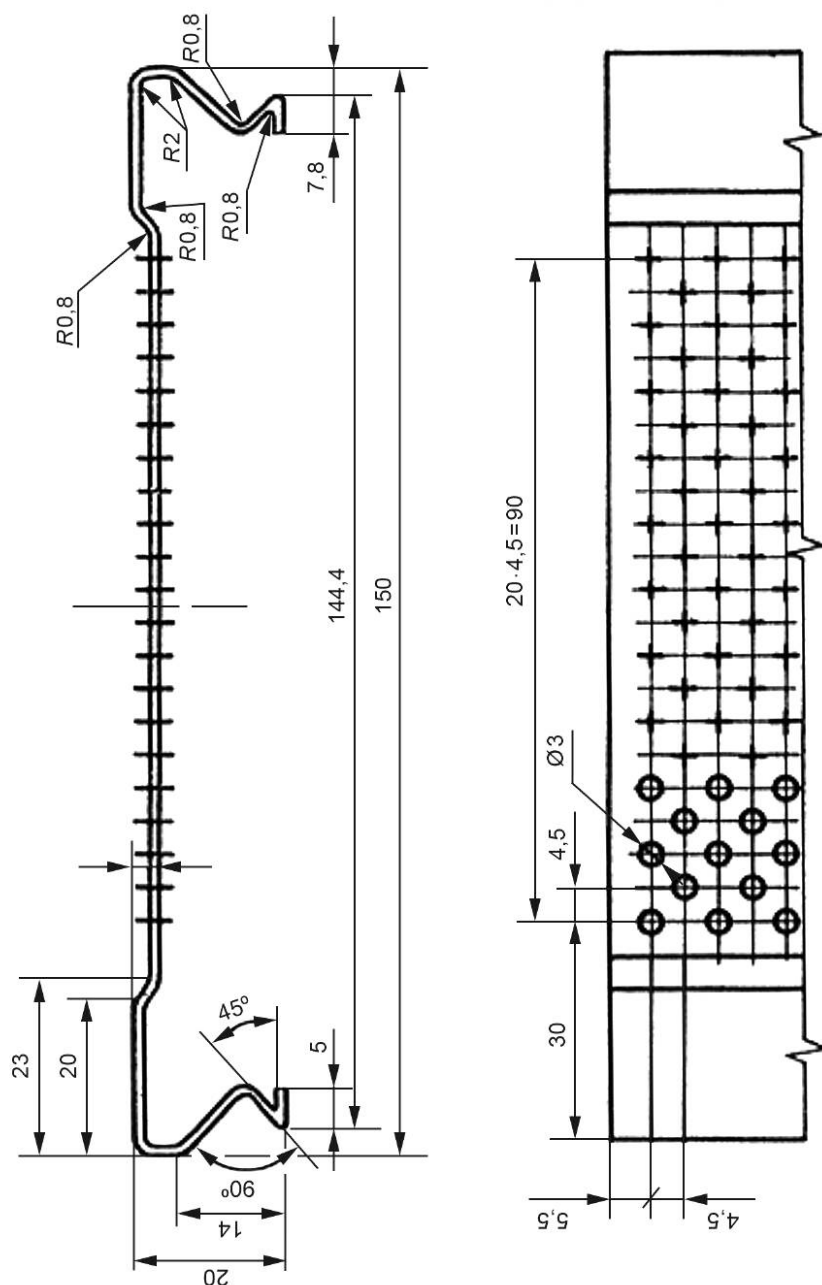
Рисунок 9 — Профили типа СА высотой 20 мм
