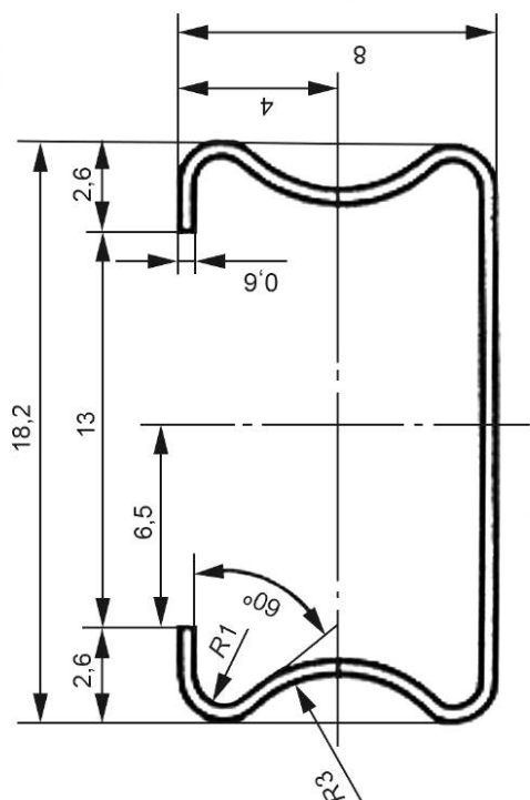
Рисунок 10 — Профили типа СА высотой 8 мм
