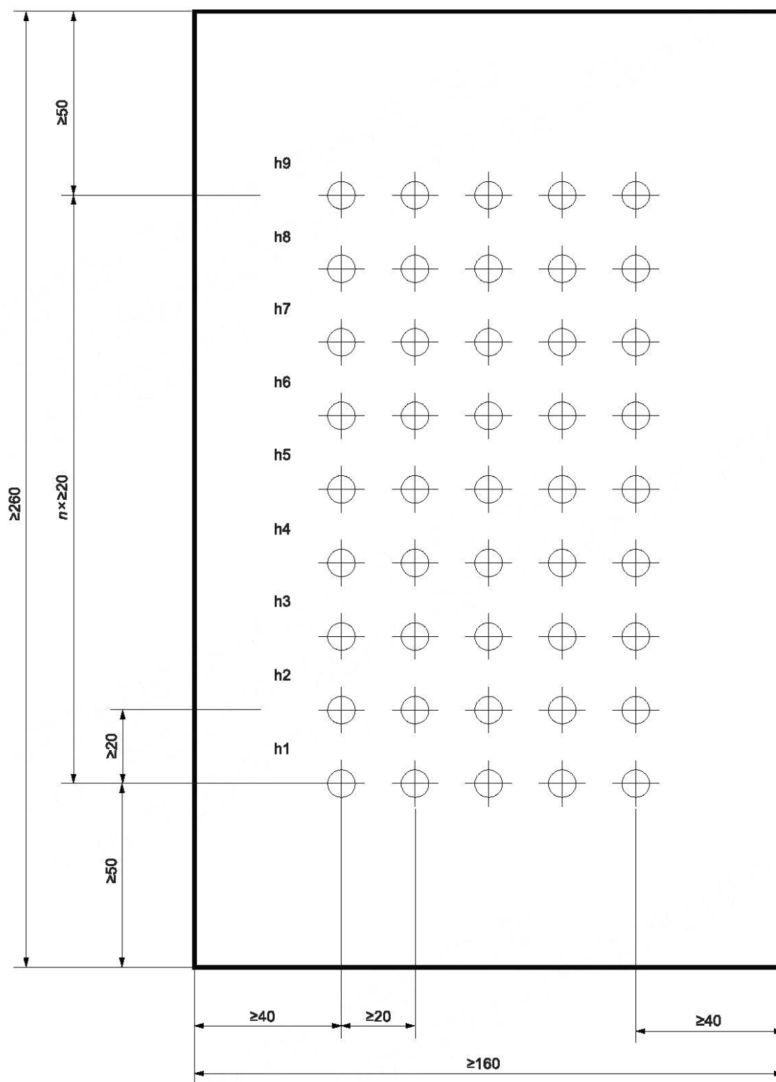
Рисунок 5 — Расположение ударов на одном испытуемом образце
