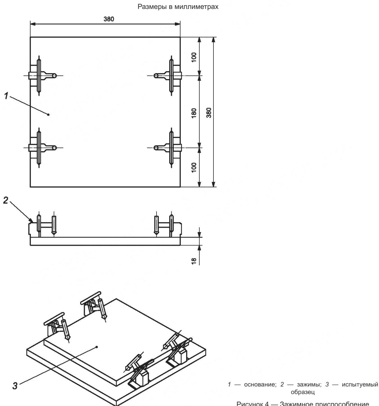
Рисунок 4 — Зажимное приспособление
