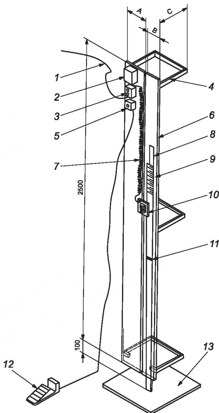
Рисунок 3 — Пример оборудования для проведения испытания при свободном падении
