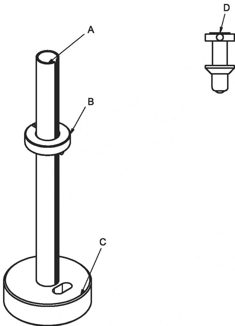
A — направляющая трубка со шкалой; B — регулируемое кольцо; C — стальное основание; D — ударник
