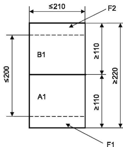
Рисунок 6 — Собранный образец для испытания для поперечной стороны
