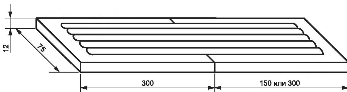
Рисунок 1 — Испытательный образец
