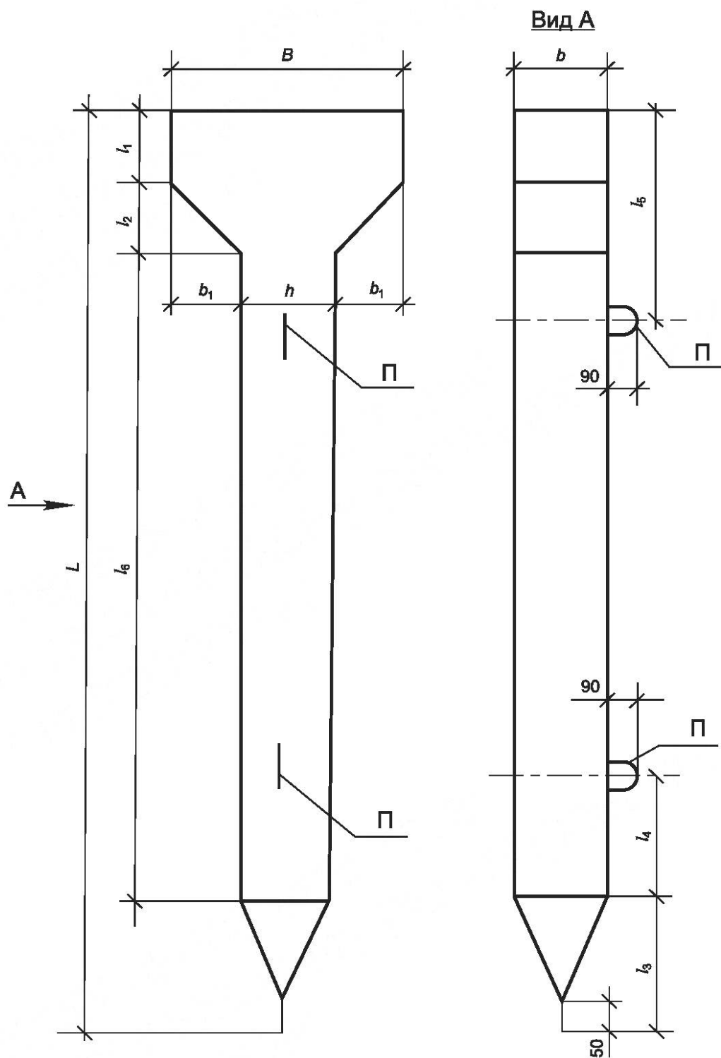
Рисунок А.1 — Колонны типа СК
