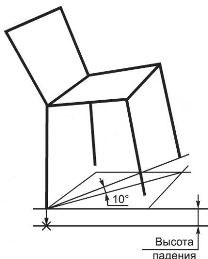
Рисунок 10 — Испытания стула на прочность при падении
