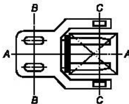
A-A — средняя вертикальная плоскость погрузчика; B-B — ведущая ось; C-C — несущая ось
