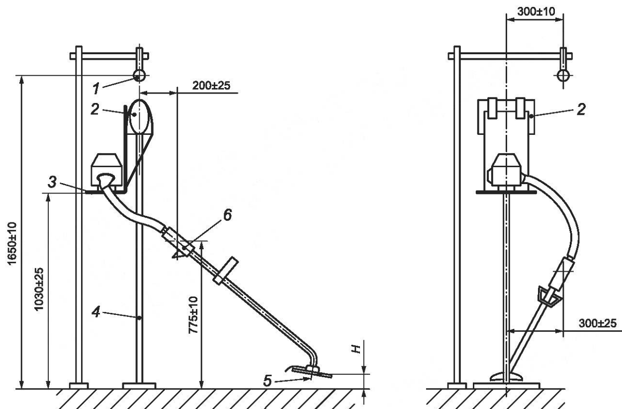
1 — микрофон (для измерений на рабочем месте оператора); 2 — узел крепления плечевых ремней; 3 — нижний край ранца; 4 — приспособление для фиксации машины; 5 — ось вращения режущего элемента; 6 — задняя рукоятка; H — высота над землей центра режущего элемента
