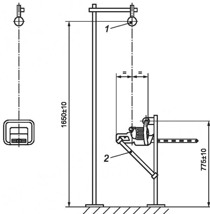
1 — микрофон (для измерений на рабочем месте оператора); 2 — приспособление для фиксации машины
