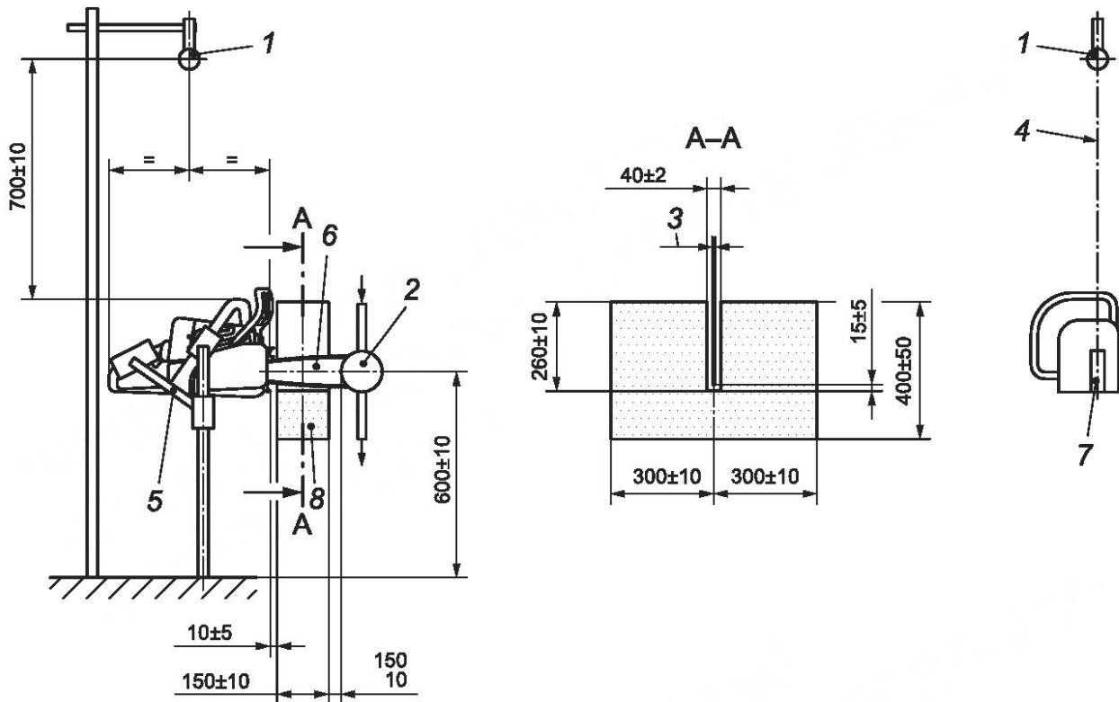
1 — микрофон (для измерений на рабочем месте оператора); 2 — нагрузочное устройство (см. пример в приложении F); 3 — ширина направляющей шины; 4 — плоскость задней рукоятки; 5 — приспособление для фиксации пилы; 6 — ось симметрии шины; 7 — задняя рукоятка; 8 — имитатор объекта обработки (деревянный брус)
