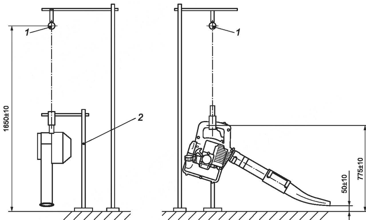
Рисунок Е.2 — Установка для испытаний воздуходувок (пылесосов) без места крепления подвеса
