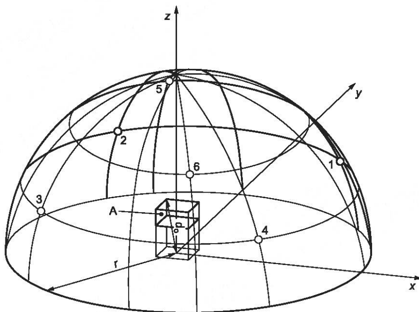
А — огибающий параллелепипед; d_0 — характеристический размер источника; r — радиус измерительной поверхности; 1,...,6 — точки измерений
