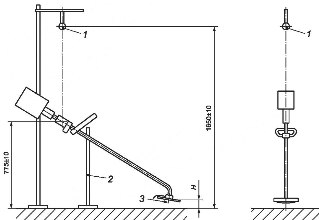
Рисунок В.1 — Установка для испытаний кусторезов и мотокос, имеющих место крепления подвеса
