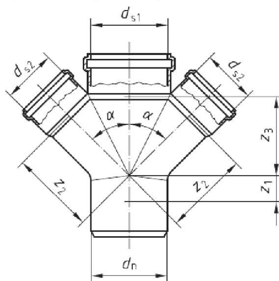
а) Крестовина
