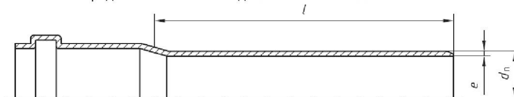
а) Труба с раструбом под уплотнительное кольцо
