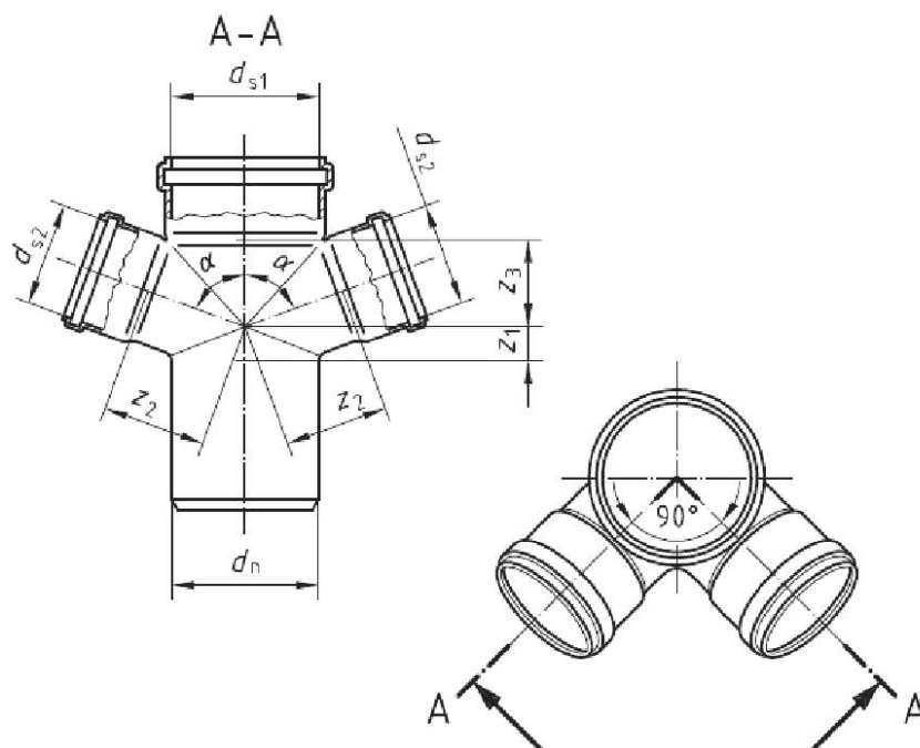
б) Крестовина двухплоскостная
