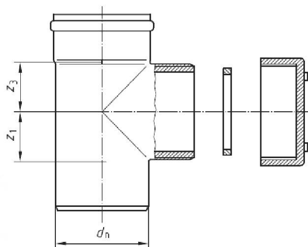
Рисунок 10 – Ревизия
