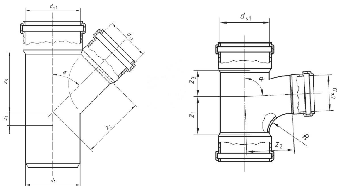
а) Тройник
