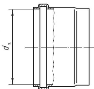
Рисунок 11 – Патрубок для стыковой сварки
