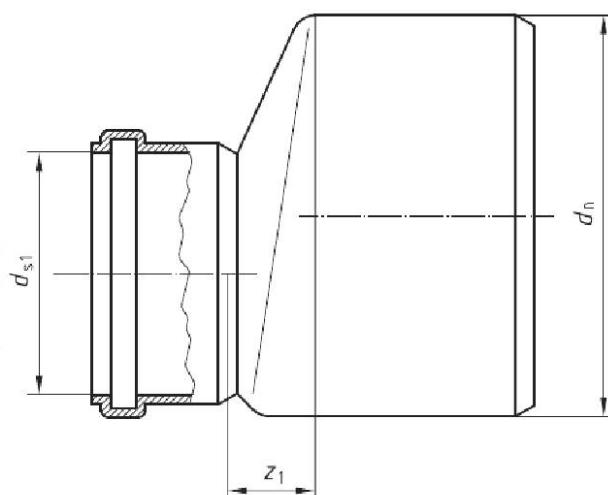
Рисунок 8 – Патрубок переходной
