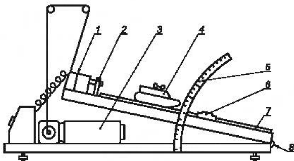
1 — микропереключатель; 2 — стопор; 3 — электромотор; 4 — носитель образца; 5 — угломерный круг; 6 — спиртовой уровень; 7 — сукно; 8 — петля
