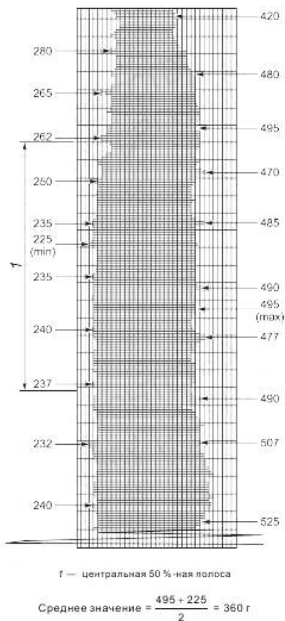
Рисунок 7 — След самописца, иллюстрирующий испытание движения двух тканей с покрытием относительно друг друга и метод построения графика значений для V_k
