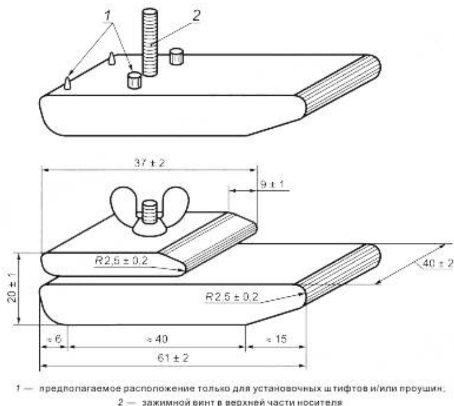
Рисунок 1 — Носитель образца для метода В
