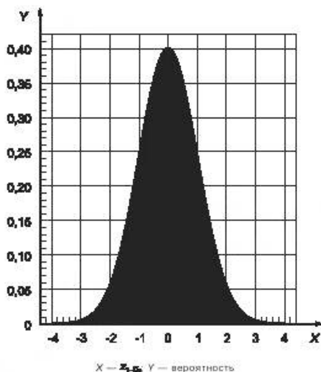
Рисунок 4 — Значения z_{1-\bar{Q}_p} для стандартного нормального распределения
