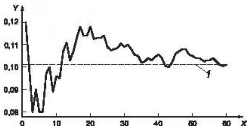
Рисунок 2 — Кумулятивное NHU (см. ISO/TR 18532)
