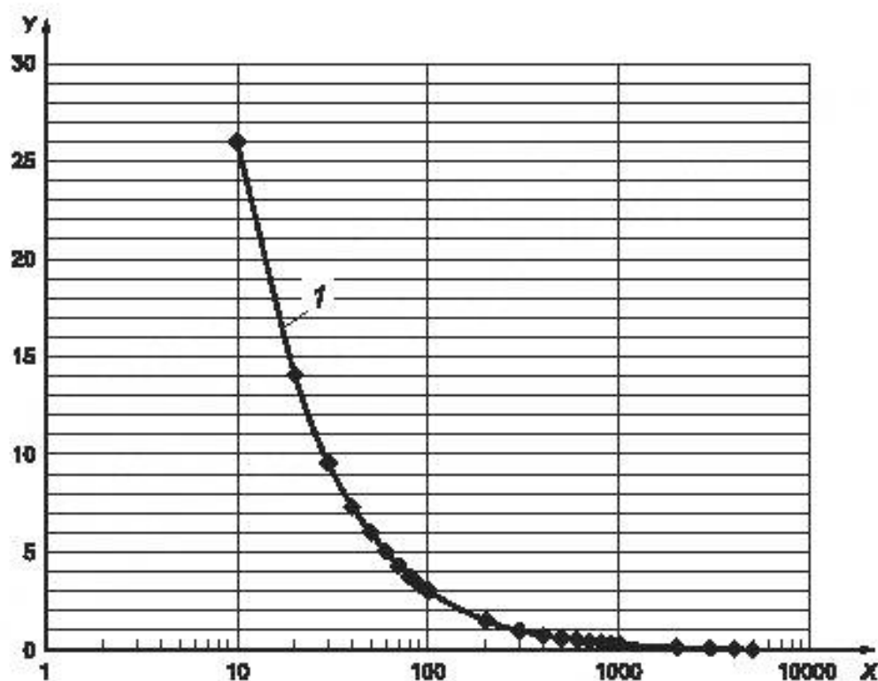
Рисунок 3 — Граница одностороннего доверительного интервала. Отсутствие несоответствующих единиц продукции и разный объем выборки n
