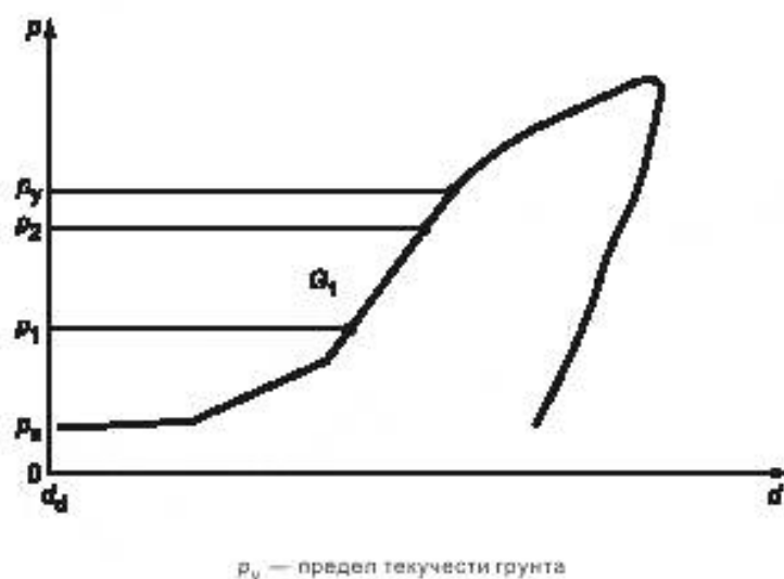
Рисунок 6 — Модуль сдвига G_1 в процедуре С
