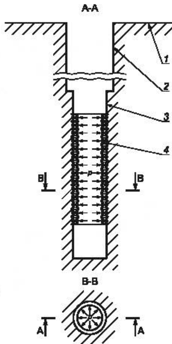
1 — поверхность земли; 2 — стенка ствола скважины; 3 — карман; 4 — расширяющийся зонд дилатометра; p — приложенное давление; А — А осевое сечение; В — В поперечное сечение
