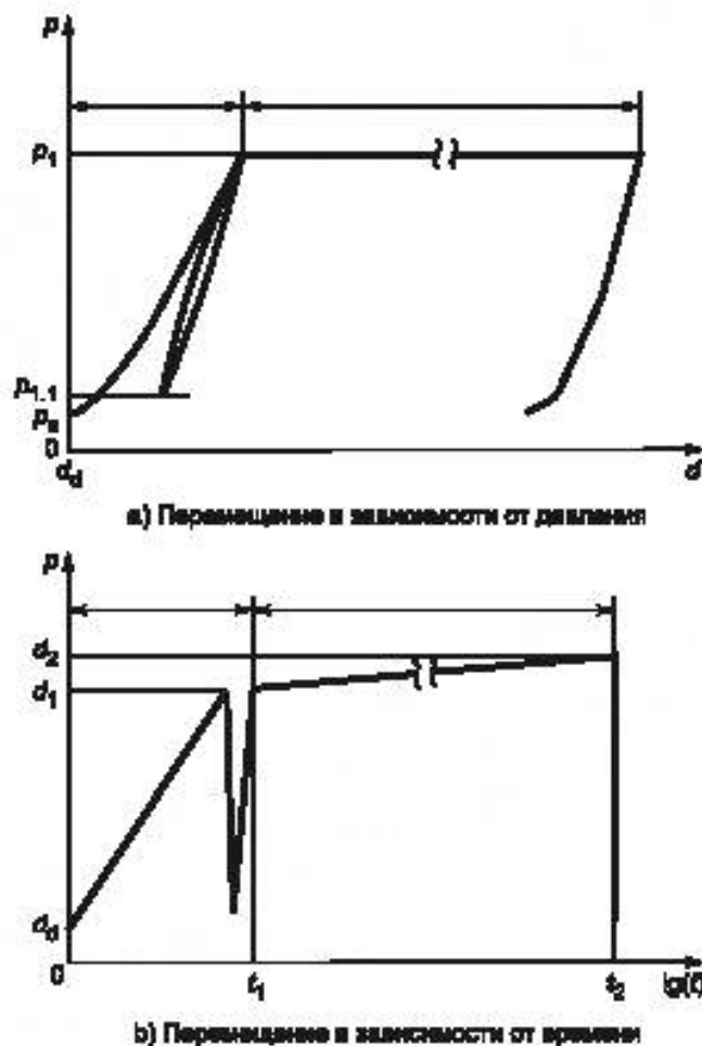
Рисунок 7 — Испытания при постоянном давлении
