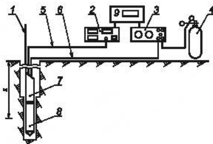
1 — установочные штанги (по отдельному заказу); 2 — блок измерения перемещения (обязательный); 3 — блок управления давлением (обязательный); 4 — источник давления (обязательный); 5 — сигнальный кабель (обязательный); 6 — нагревательный трубопровод (обязательный); 7 — труба для сбора отложений (по отдельному заказу); 8 — регистратор данных (по отдельному заказу); z — глубина испытания
