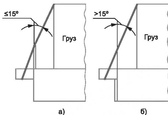
Рисунок 1 — Допускаемые положения проволочных растяжек, обвязок относительно бортов платформы
