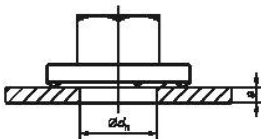
Рисунок 2 — Присоединительные размеры (гайки еще не приварены)
