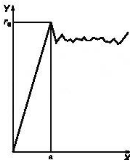
Рисунок 4 — Типичный пример записанного графика F_S , имеющего пик
