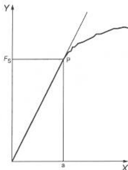
Рисунок 5 — Типичный пример записанного графика F_S , не имеющего пиков
