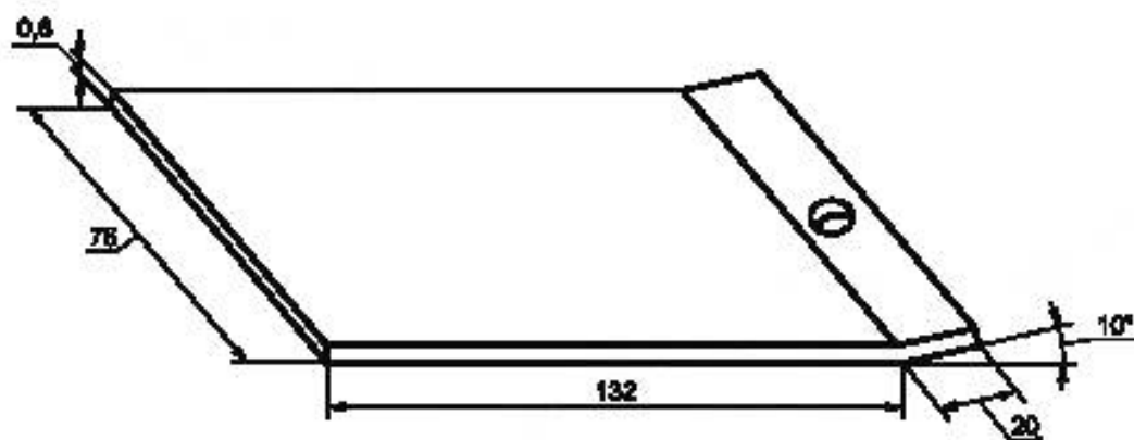
Рисунок 2 — Испытательная металлическая пластина
