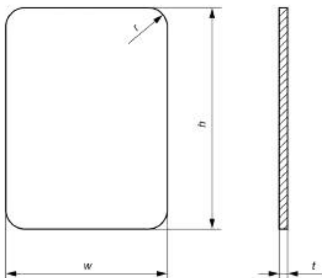
Рисунок 1 — Размеры стекол для прямоугольных окон
