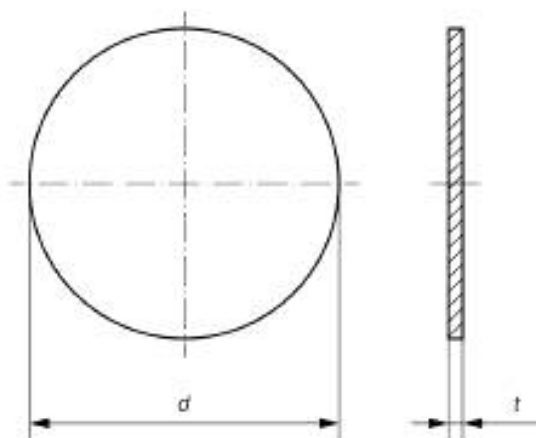
Рисунок 2 — Размеры стекол для бортовых иллюминаторов
