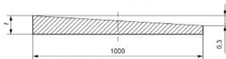
Рисунок 4 — Разнотолщинность стекла
