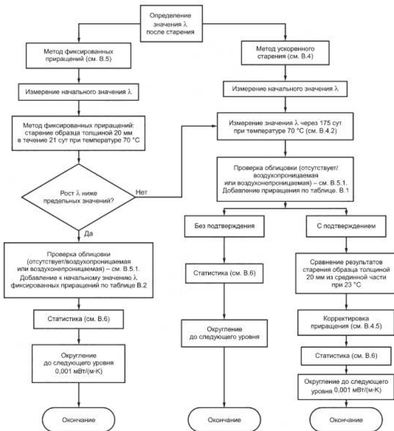
Рисунок В.1 — Блок-схема альтернативных методов старения
