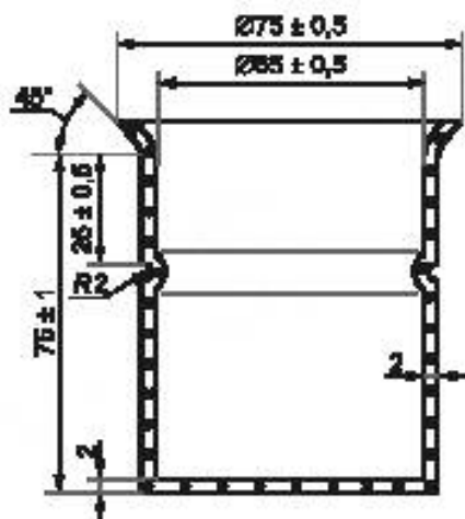
Рисунок А.3 — Пример стакана для испытания
