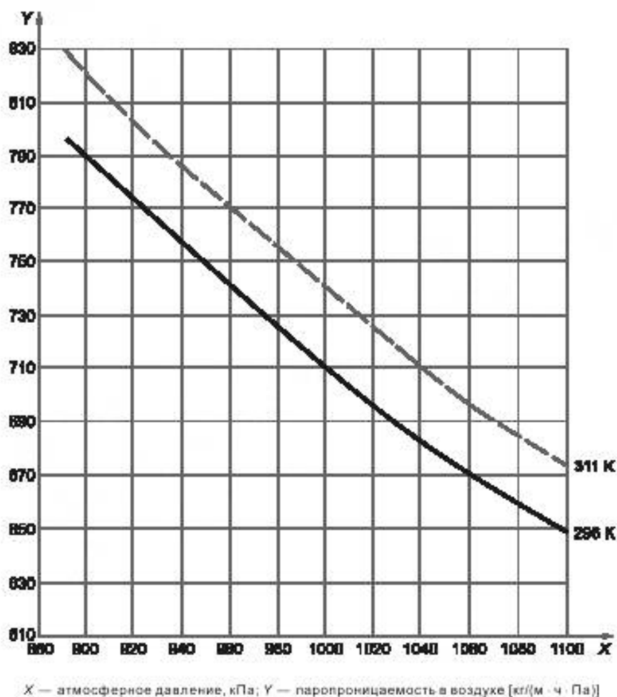
Рисунок В.1 — Зависимость паропроницаемости в воздухе от атмосферного давления в соответствии с формулой (В.4) при температурах 23 °С (296 К) и 38 °С (311 К)
