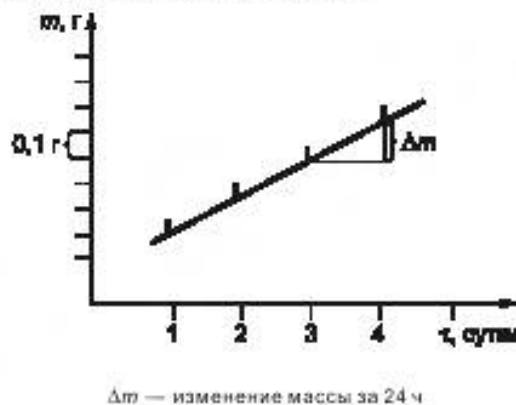
Рисунок 3 — График зависимости изменения массы от времени
