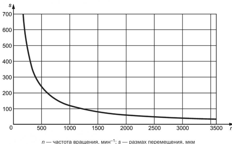
Рисунок D.1 — Изменение составляющей перемещения на частоте вращения ротора при ее уменьшении с сохранением постоянного среднеквадратичного значения скорости вибрации 4,5 мм/с
