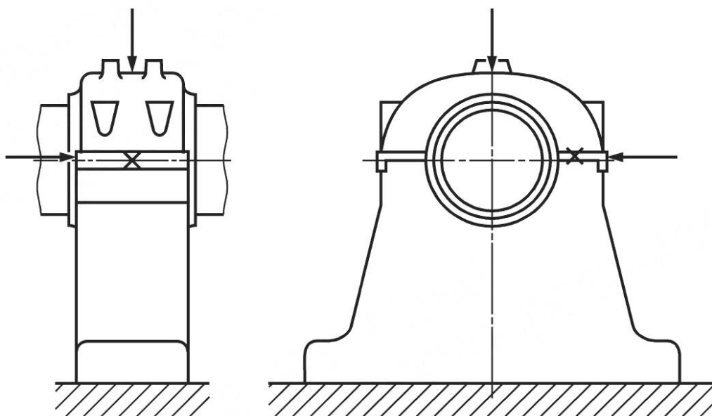
Рисунок 1 — Точки измерений на опорах/крышках подшипников
