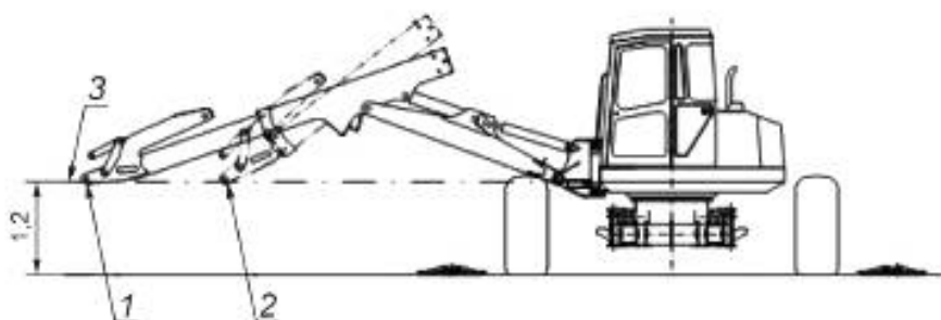
Рисунок 2 — Определение опрокидывающей нагрузки вперед/назад
