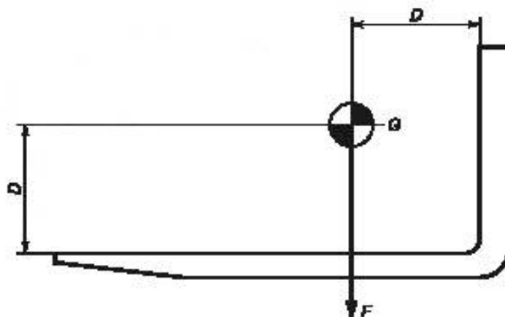
Рисунок 1 — Расстояние центра нагрузки для вилочного оборудования
