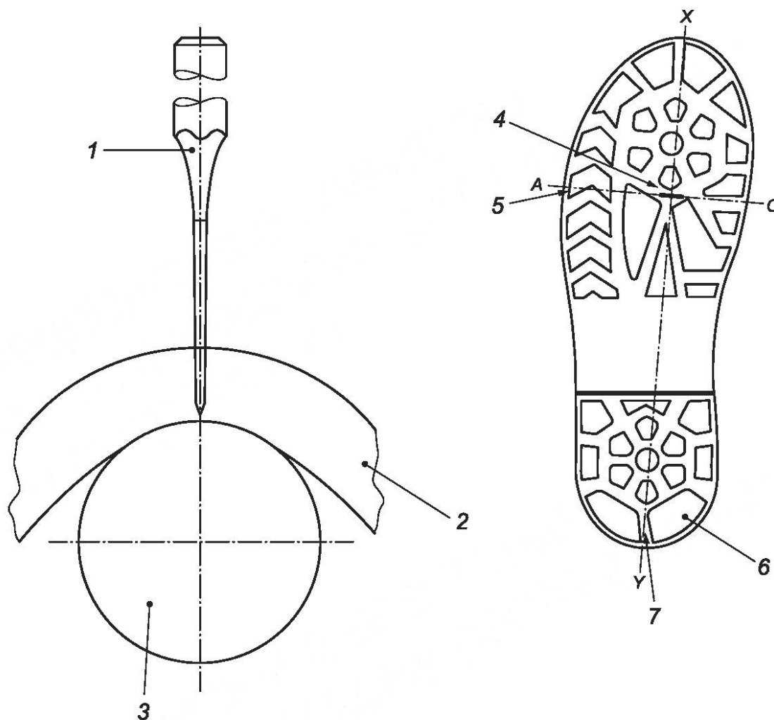
1 — режущий инструмент; 2 — испытуемая проба; 3 — оправка испытательной машины, радиус 15 мм; 4 — одиночный надрез на линии максимального напряжения; 5 — вспомогательная линия AC, параллельна или на линии максимального напряжения; 6 — выступы протектора; 7 — продольная ось XY
