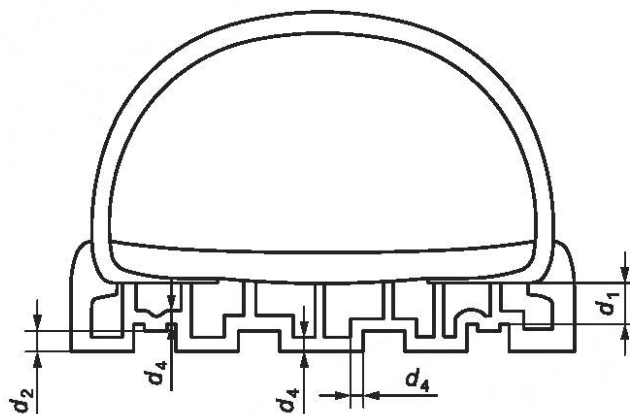
Рисунок 40 — Обувь клеевого метода крепления (минимальная толщина)
