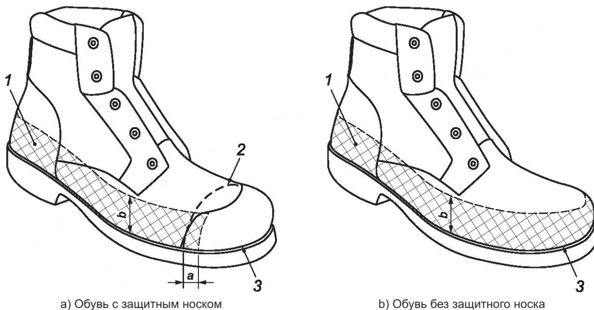
1 — подлежащая испытанию область перекрытия защитного носка; 2 — задний край защитного носка; 3 — линия кромки; a — перекрытие защитного носка/защитной области, мм; b — высота защищаемой области, мм
