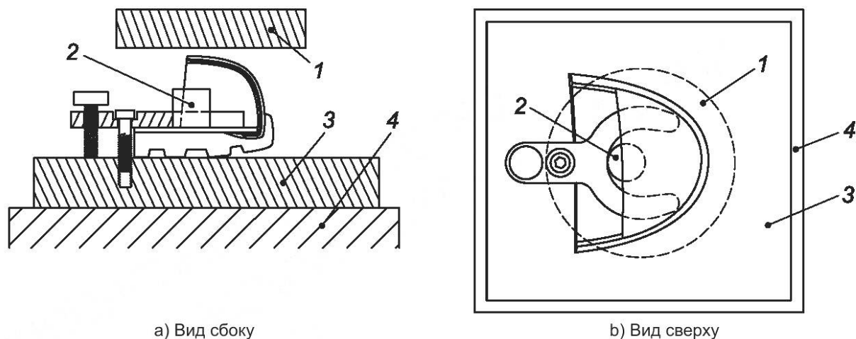
а) Вид сбоку 1 — верхняя пластина; 2 — цилиндр из глины для лепки; 3 — зажимное устройство; 4 — нижняя пластина
