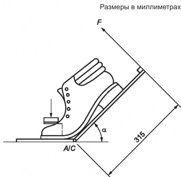
A/C — линия изгиба; F — усилие (30 \pm 0,5) Н; \alpha — угол изгиба
