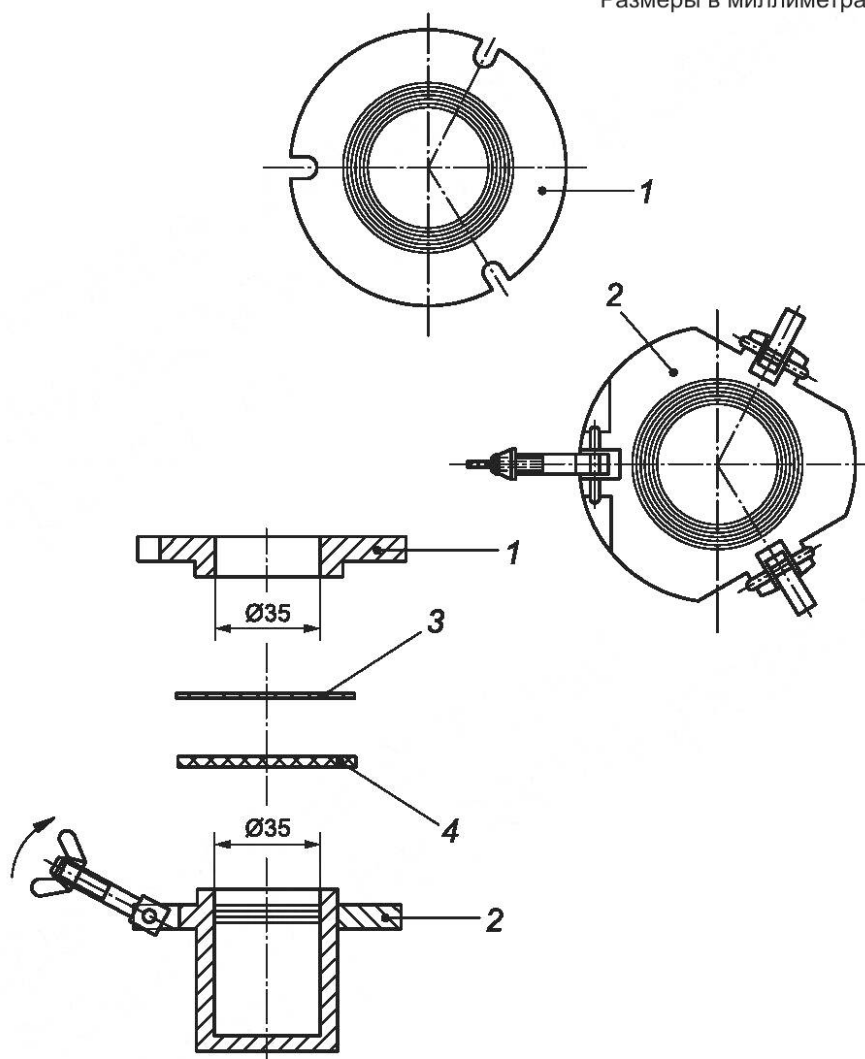
1 — верх; 2 — низ; 3 — изоляционная прокладка; 4 — испытуемая проба
