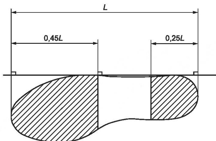
Рисунок 36 — Область протектора
