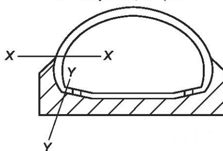
Тип b — Стандартная затыжка, подошва без выступающего края
