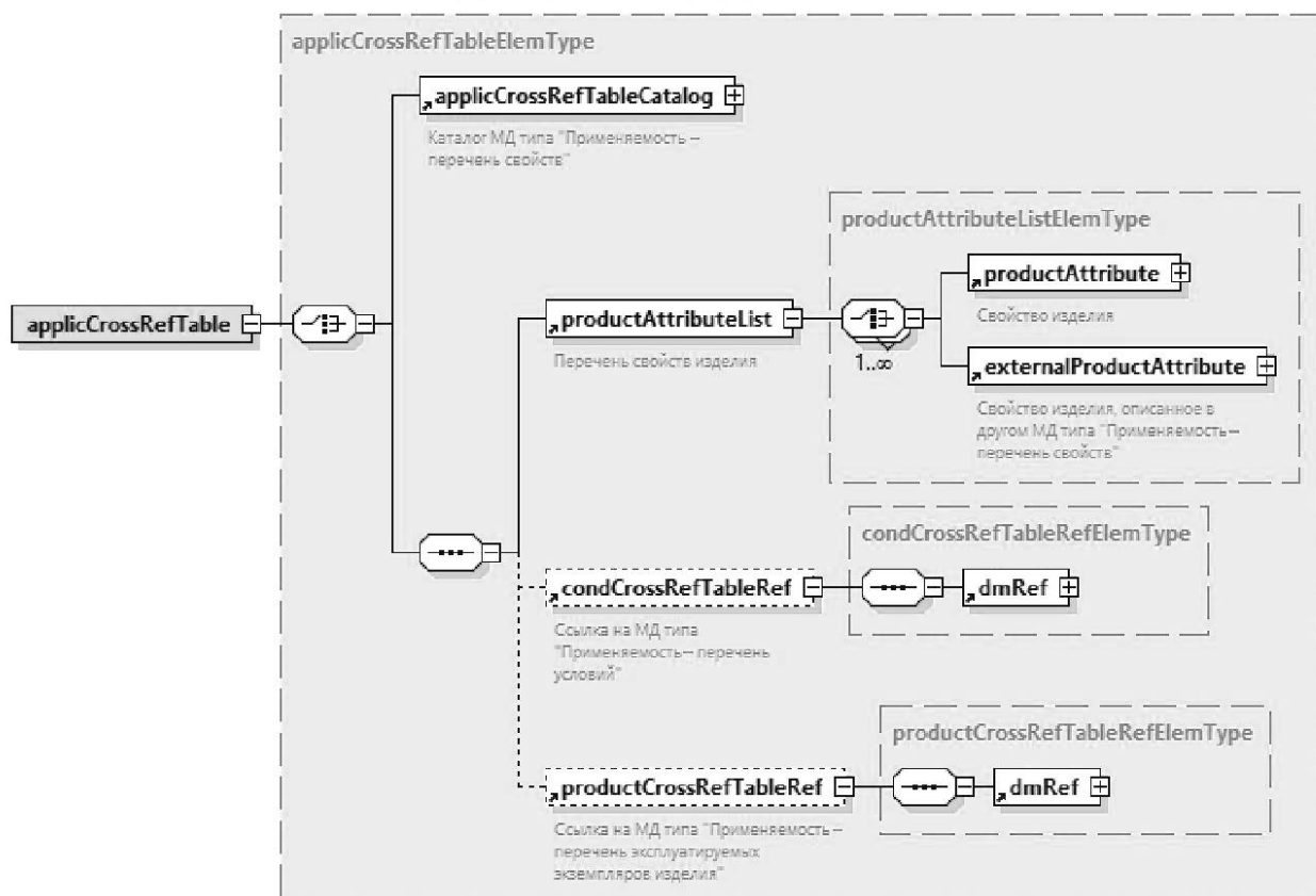
Рисунок А.38 — Схема элемента &lt;applicCrossRefTable&gt;
