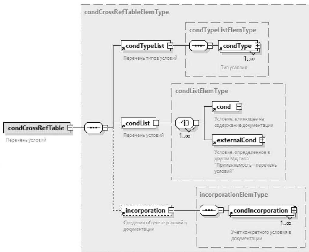
Рисунок А.40 — Схема элемента &lt;condCrossRefTable&gt;
