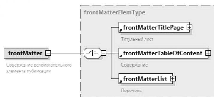
Рисунок А.47 — Схема элемента <frontMatter>
