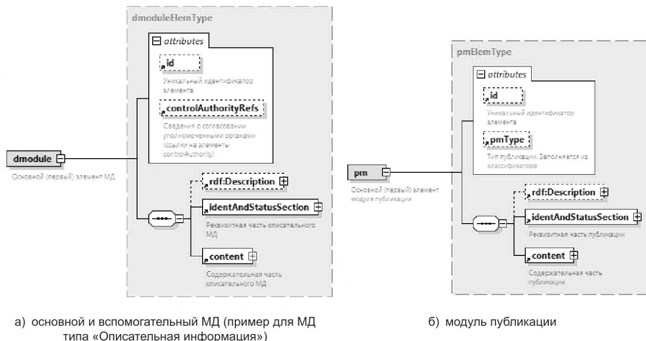
Рисунок A.1 — Верхнеуровневая структура МД
