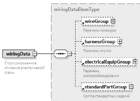
Рисунок А.35 — Схема элемента &lt;wiringData&gt;
