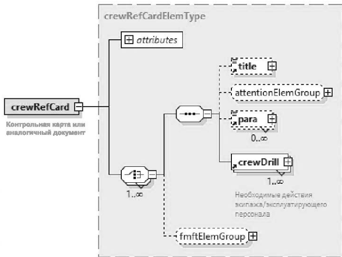
Рисунок А.32 — Схема элемента <crewRefCard>
