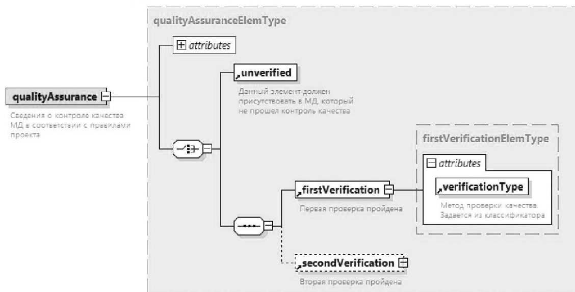
Рисунок А.11 — Схема элемента &lt;qualityAssurance&gt;
