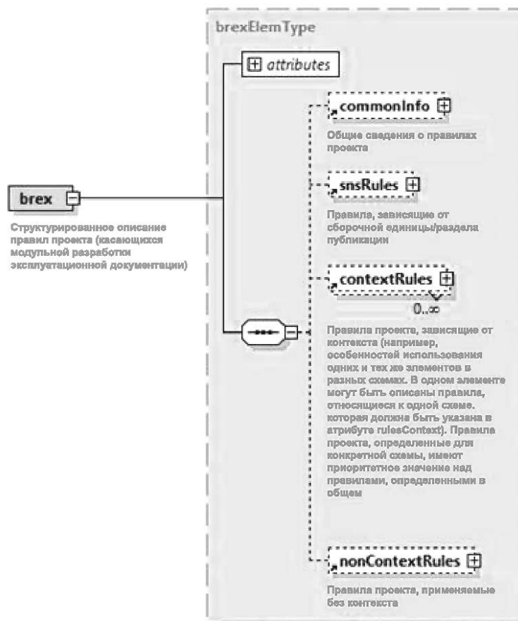
Рисунок А.46 — Схема элемента <brex>
