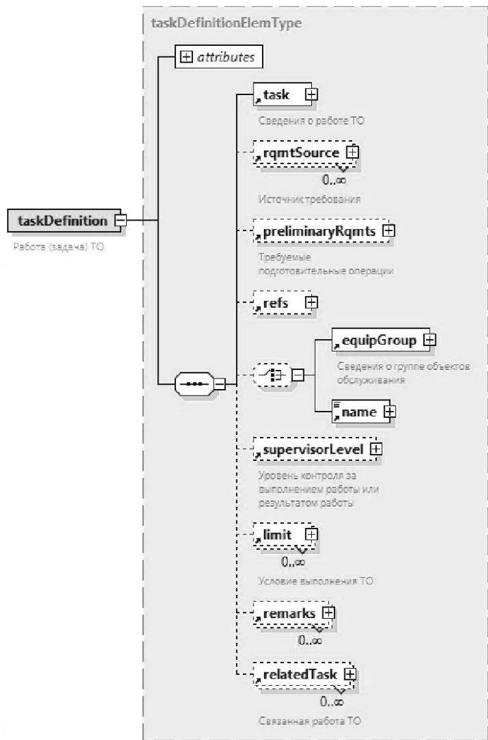
Рисунок А.24 — Схема элемента <taskDefinition>
