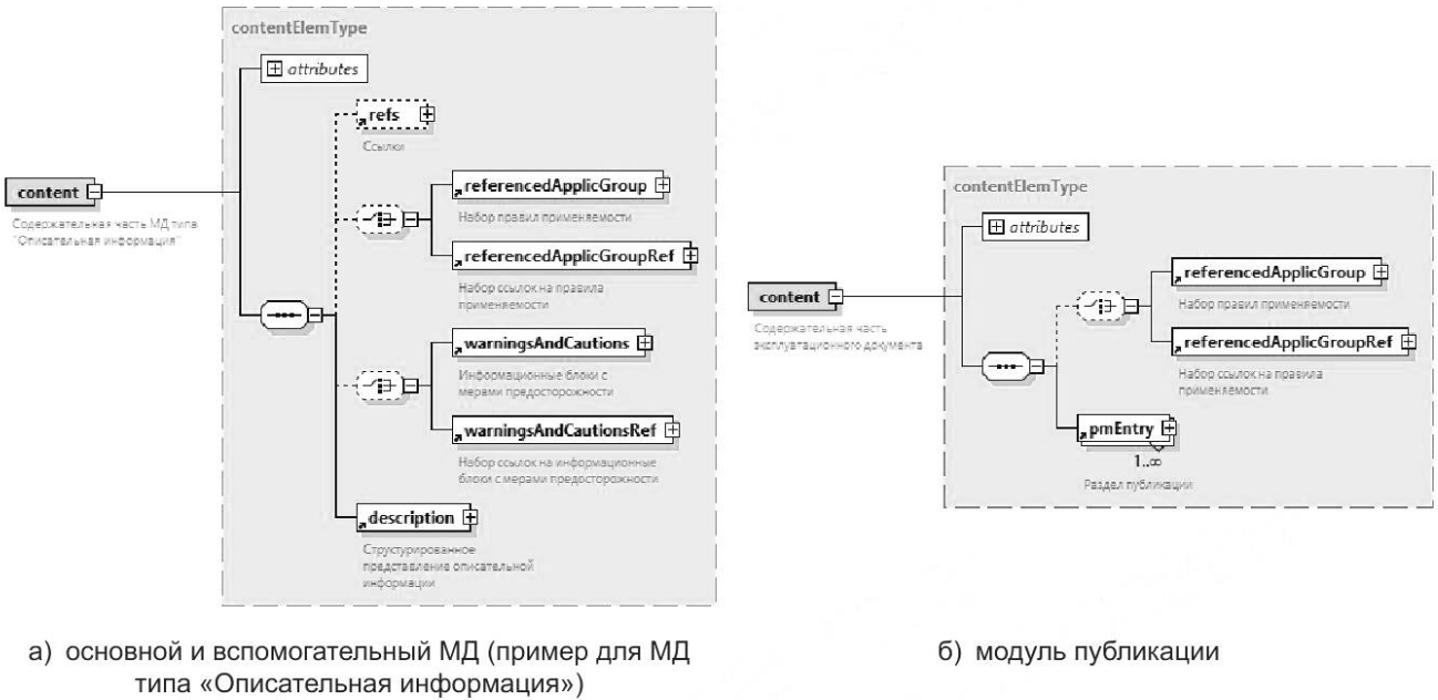
Рисунок А.5 — Структура содержательной части модуля данных
