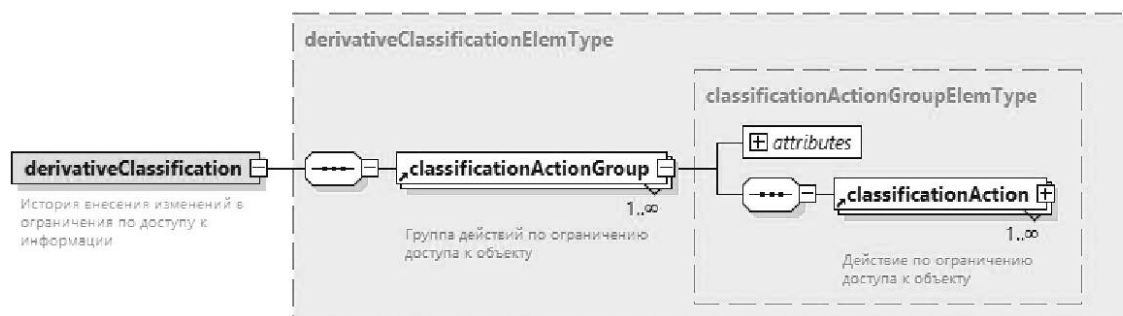
Рисунок А.10 — Схема элемента &lt;derivativeClassification&gt;
