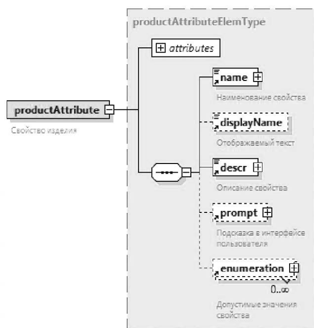
Рисунок А.39 — Схема элемента &lt;productAttribute&gt;
