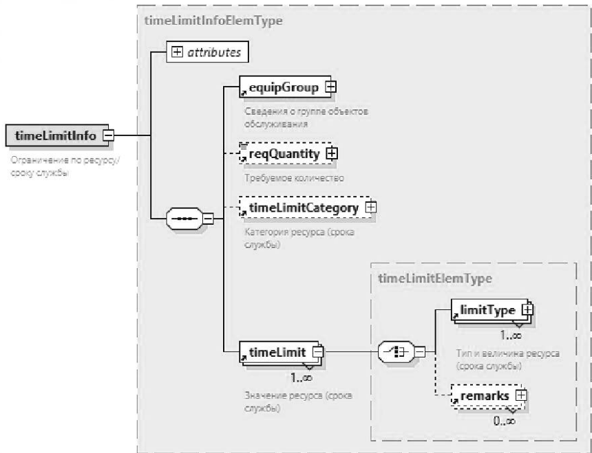
Рисунок А.25 — Схема элемента <timeLimitInfo>
