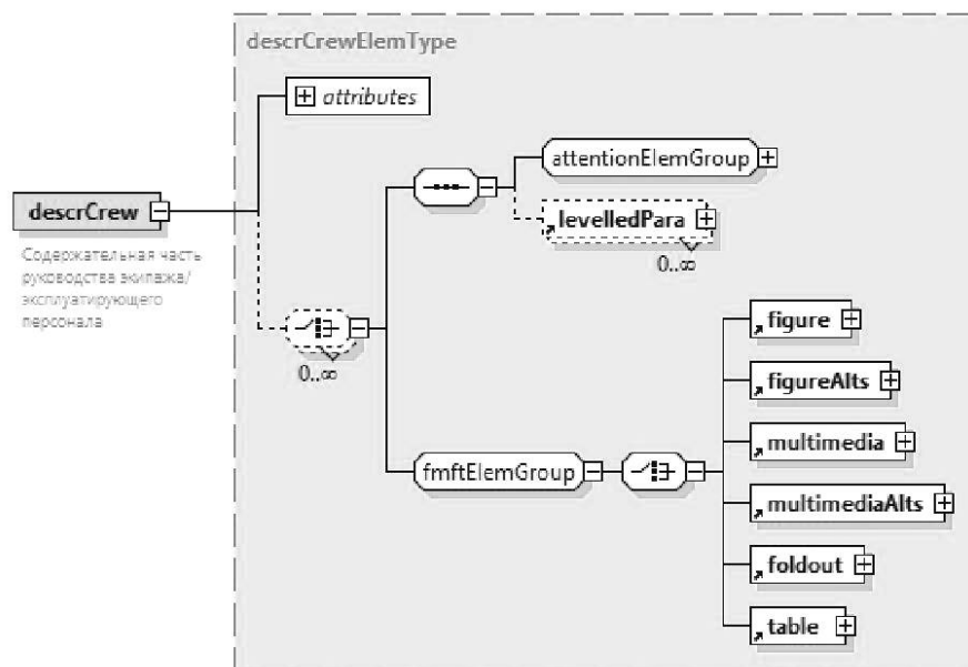
Рисунок А.34 — Схема элемента &lt;descrCrew&gt;
