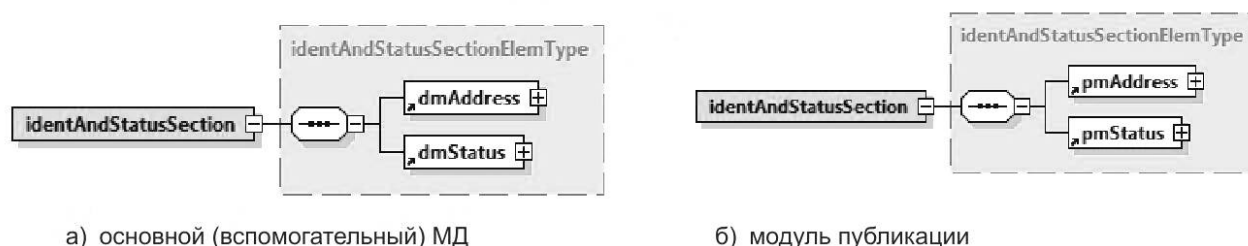
Рисунок A.2 — Верхнеуровневая структура РЧ МД
