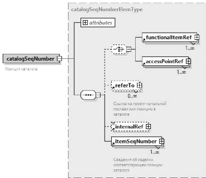
Рисунок А.21 — Схема данных элемента <catalogSeqNumber>
