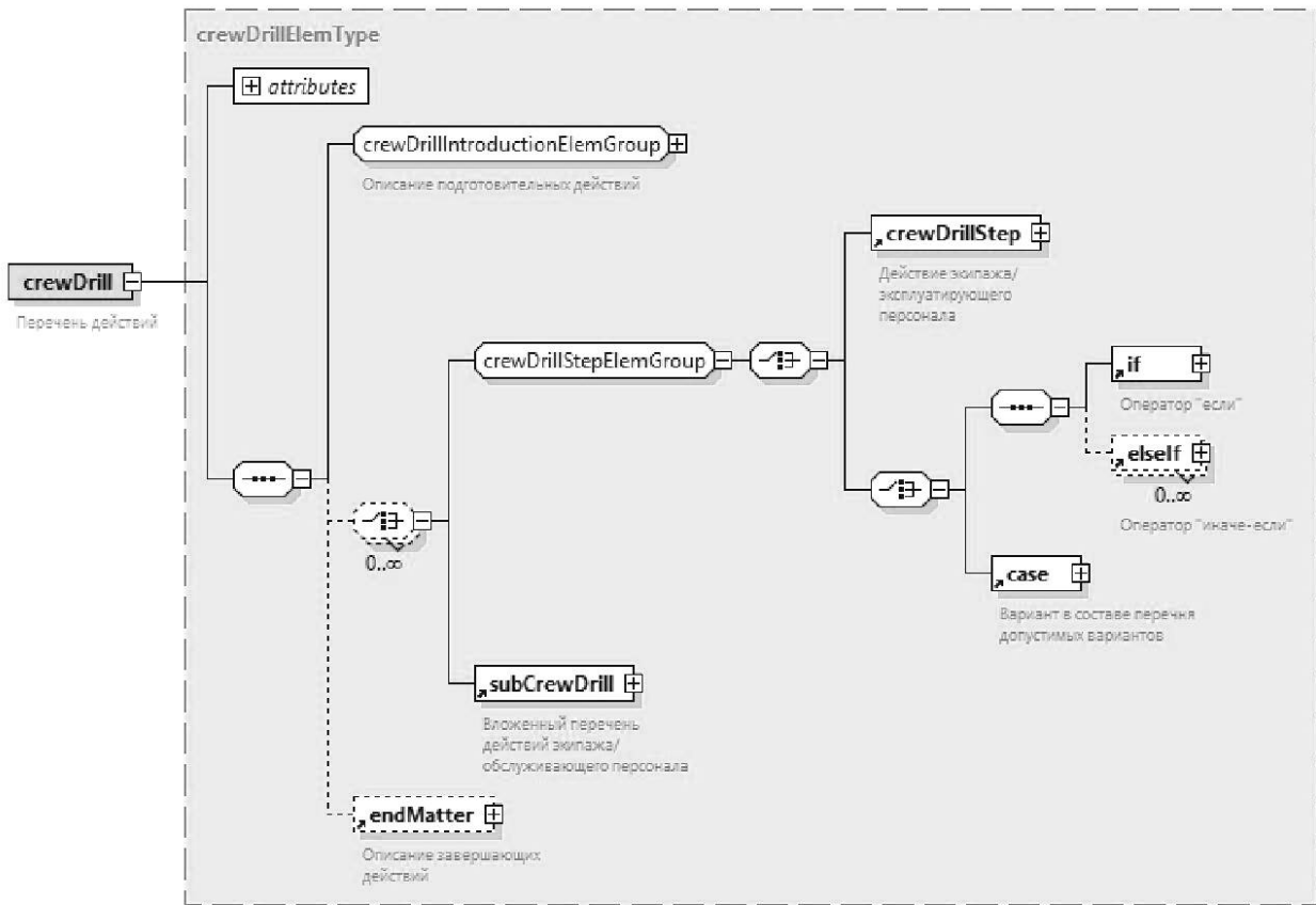
Рисунок А.33 — Схема элемента <crewDrill>
