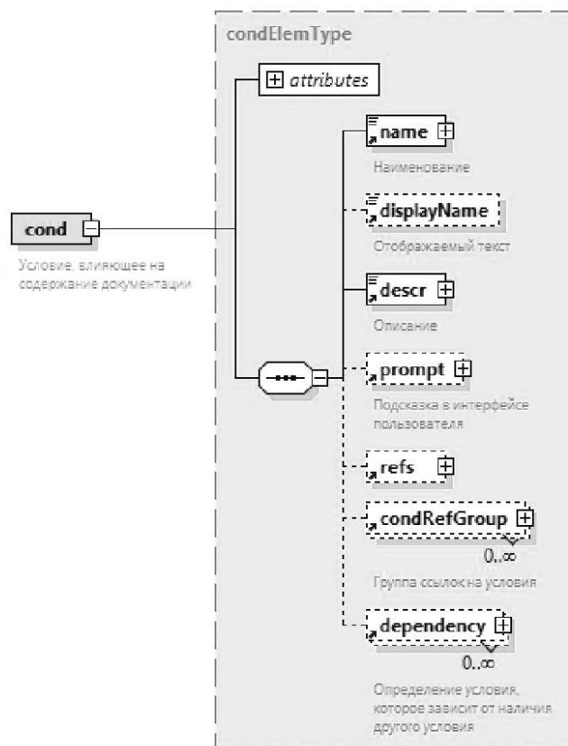
Рисунок А.41 — Схема элемента &lt;cond&gt;
