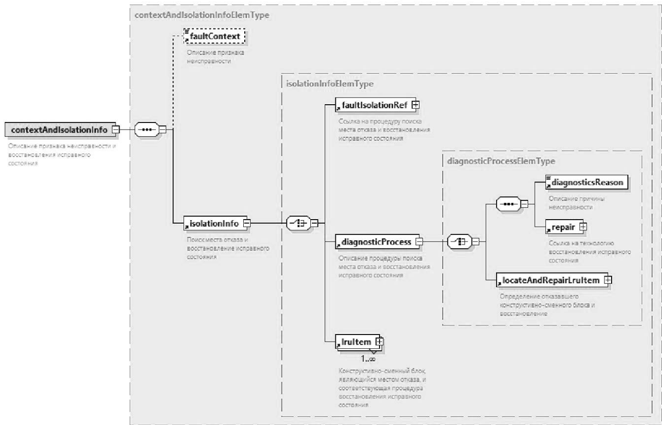
Рисунок А.30 — Схема элемента <contextAndIsolationInfo>
