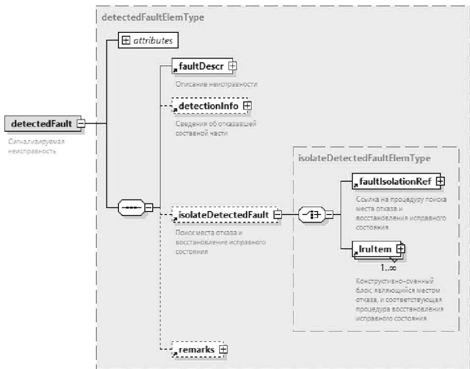
Рисунок А.29 — Схема элемента <detectedFault>
