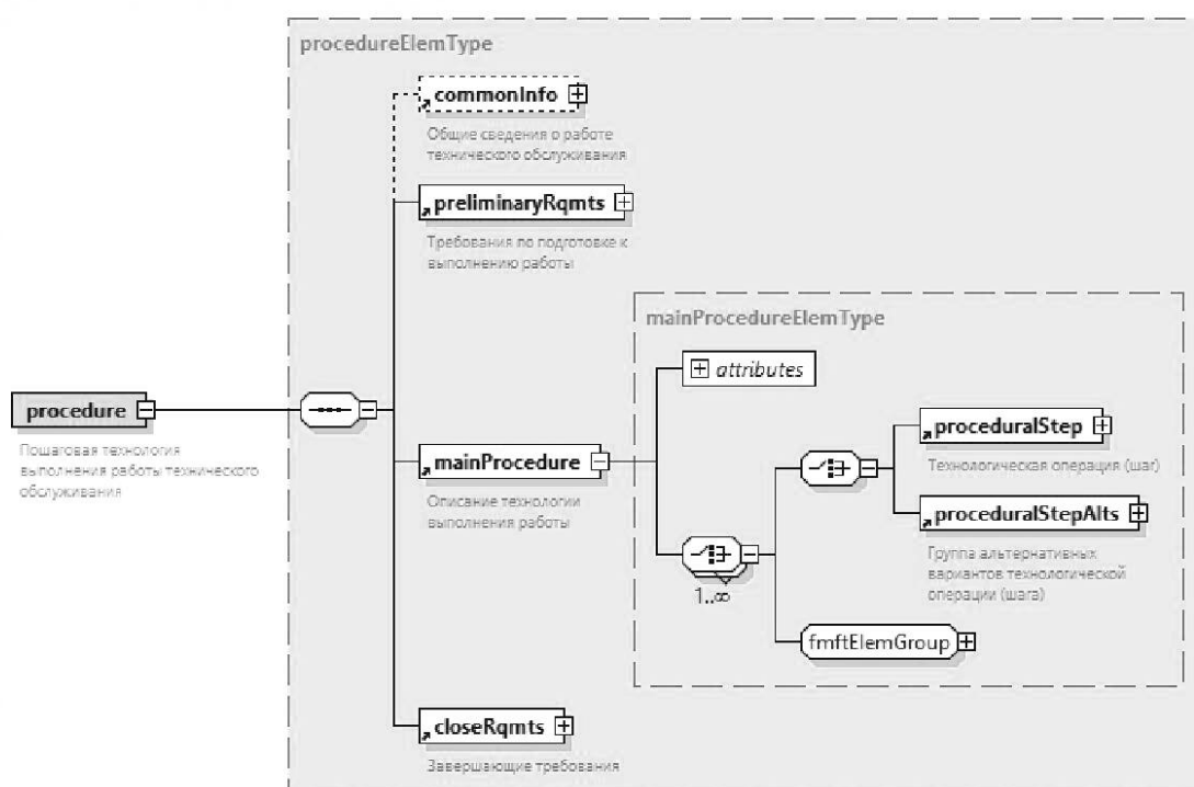
Рисунок А.26 — Схема элемента <procedure>
