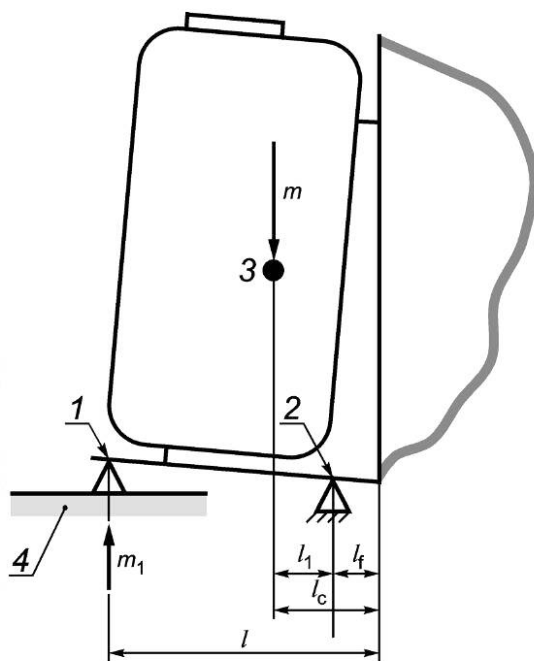
1 — точка взвешивания; 2 — зафиксированная точка; 3 — центр тяжести; 4 — весы по 4.7 а); l_1 — расстояние от точки взвешивания 1 до зафиксированной точки 2; l_f — расстояние между вертикальной плоскостью, проходящей через точки крепления лямок до зафиксированной точки
